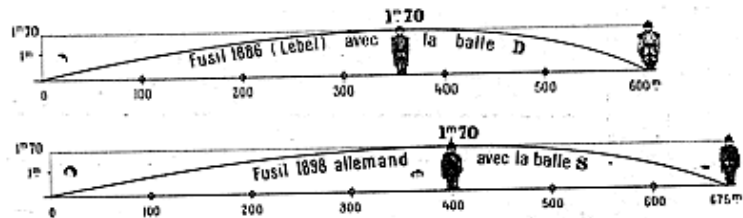
Fig. f.--Zones dangereuses du fusil français avec la balle D. du fusil allemand avec la balle S.
