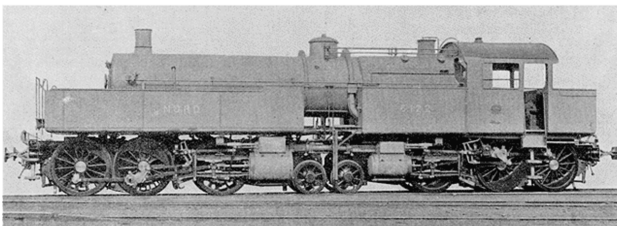
Nouvelle locomotive «de force», à seize roues, mise en service par la Compagnie du Nord.
