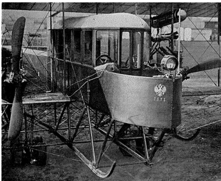
La cabine, pour dix personnes, du biplan géant de l'ingénieur russe Sikorsky.
