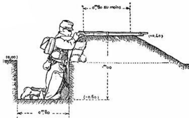
Tranchée pour tireur à genoux.
