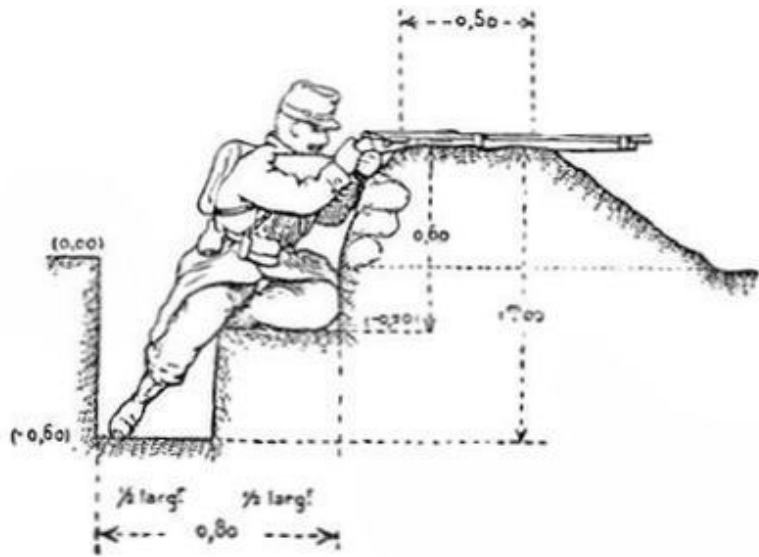
Tranchée pour tireur assis
