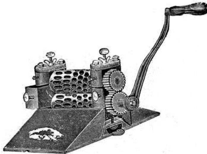
Fig. 12½.
