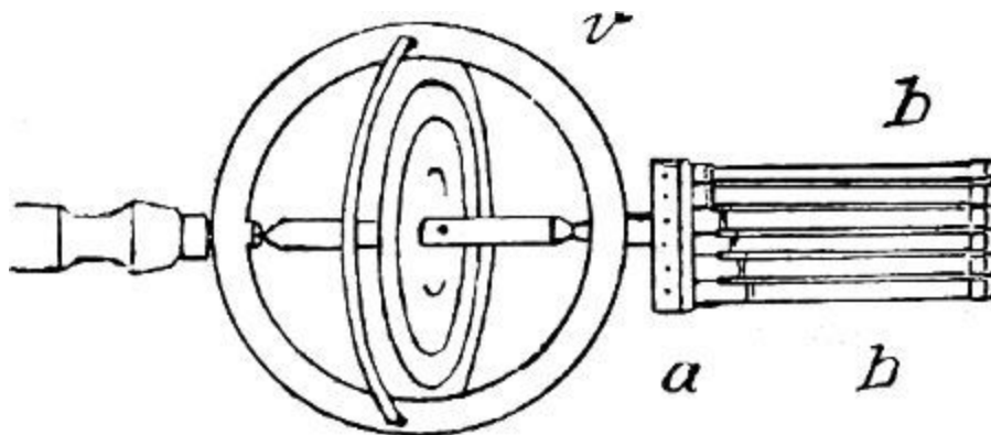
Frahm'scher Kreisel. Aus Neesen: Hörbare Strahlen.
