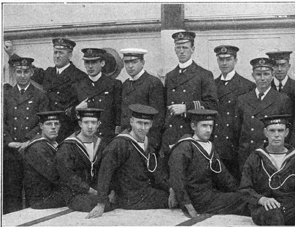
Shackleton.
