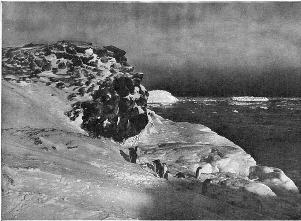
Poollandschap.
