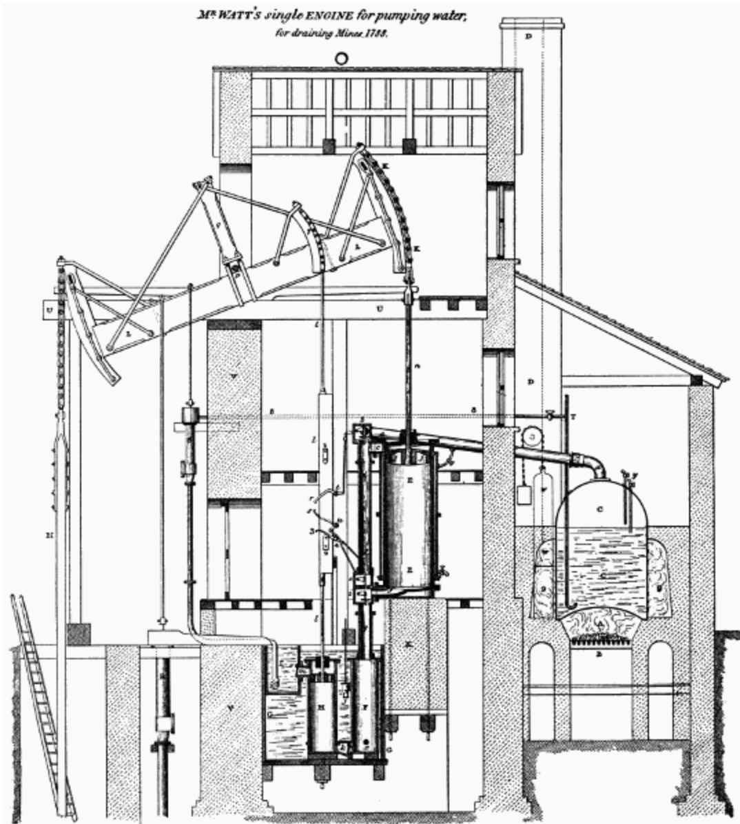
Abb. 15. Watts einwirkende Dampfmaschine 1788. (Nach Farey.)
