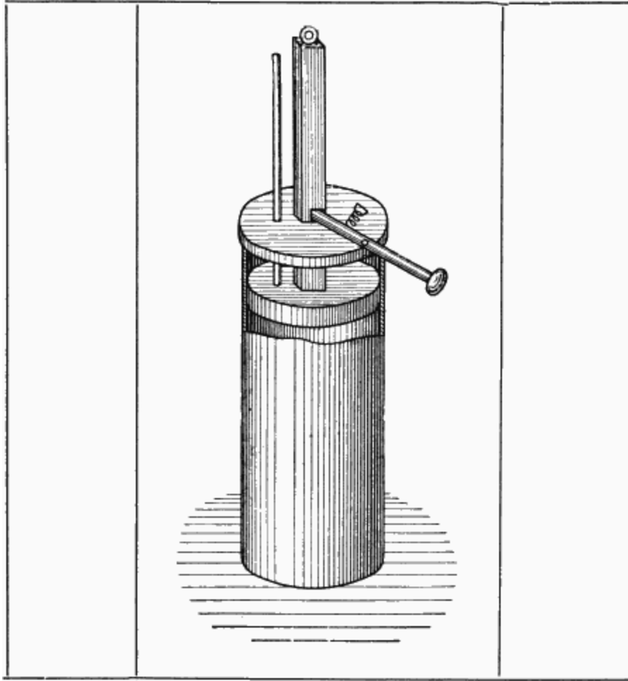
Abb. 6. Papins atmosphärische Kolbenmaschine 1690.
