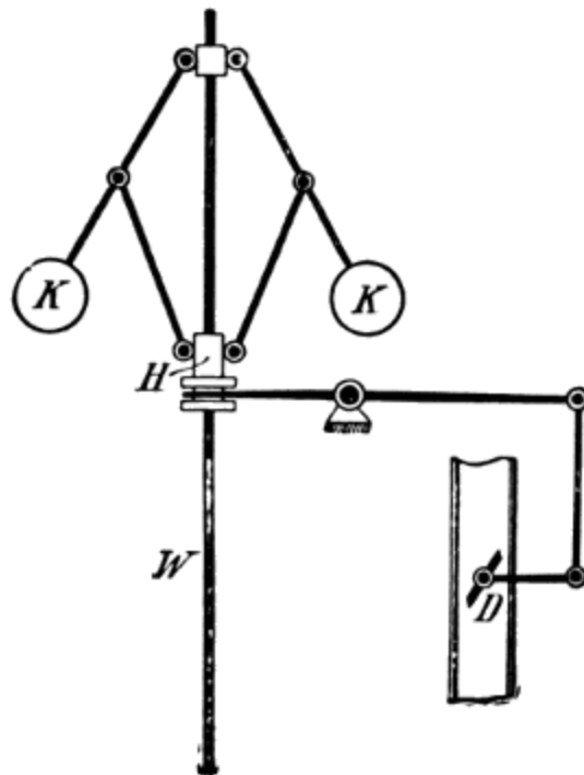
Abb. 20. Regulator.
