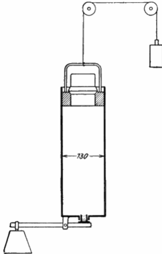
Abb. 5. Papins Pulvermaschine 1688.
