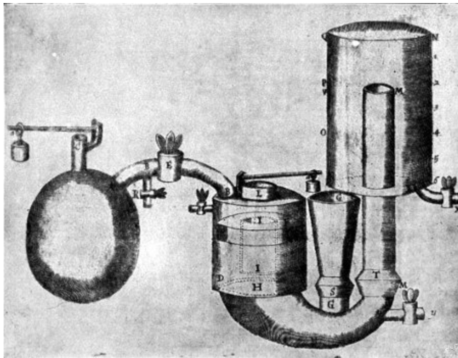
Abb. 8. Papins Dampfpumpe 1707.
