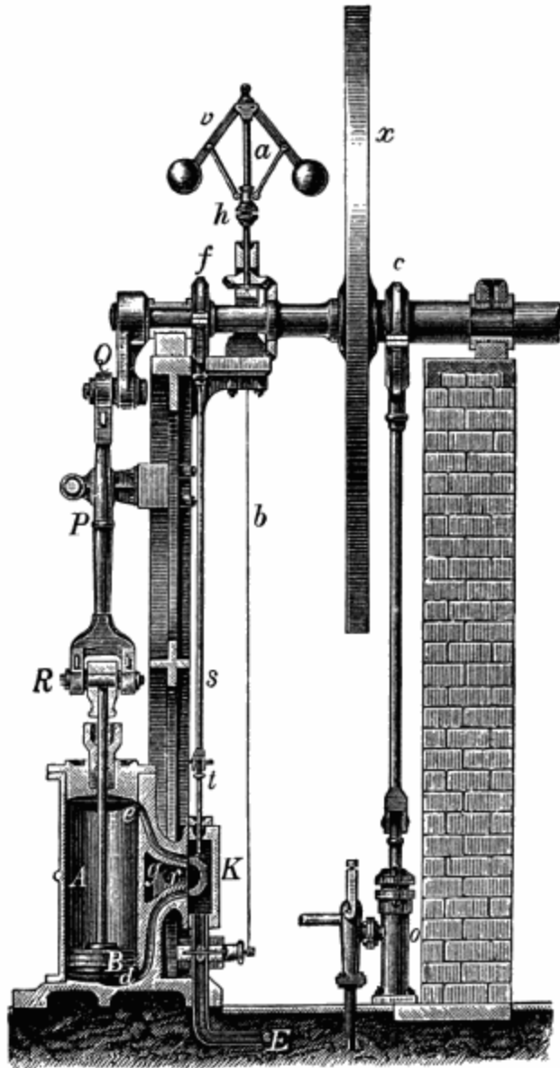
Abb. 22. Hochdruckmaschine, wie sie erst nach Watt gebaut wurde, vertikale Einzylindermaschine. E Dampfweg vom Kessel nach dem Dampfverteilungsbehälter oder Schieberkasten \kappa , zwischen E und \kappa die Drosselklappe. A Dampfzylinder, e und d lassen den Dampf ein und aus, der entweichende Dampf geht durch g und r ins Freie. B Kolben, R Kreuzkopf, P Pleuel- (oder Kurbelstange), Q Kurbelzapfen, f Exzentrerscheibe, auf der durch Q gedrehten Welle sitzend, die auch das Schwungrad x dreht, die Exzentrerscheibe bewegt den Dampfschieber in \kappa auf und ab; h a v Regulator, hochgehendes h hebt b und dreht die Drosselklappe zwischen \kappa und E. c Exzentrerscheibe, betätigt
