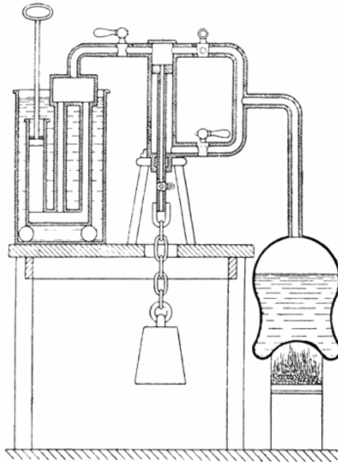
Abb. 13. Watts erstes Modell einer Dampfmaschine mit getrenntem Kondensator 1765. (Aus »Zeitschr. d. Vereins D. Ingenieure« 1896, S. 979.)
