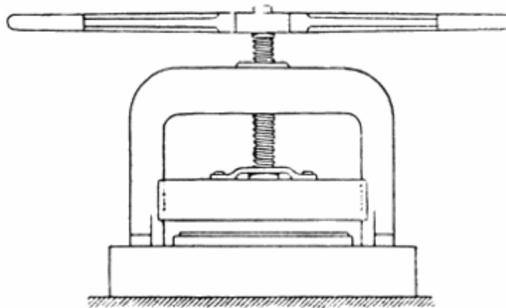
Abb. 23. Kopierpresse (Zeitschr. d. Ver. D. Ing. 1896.)
