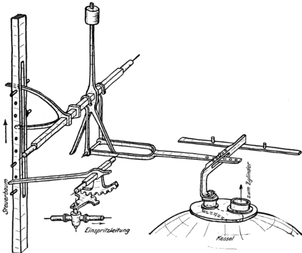
Abb. 10. Beightons Steuerung 1718.
