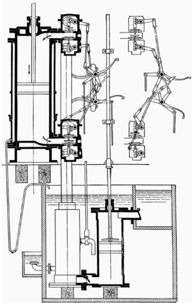
Abb. 17. Zylinder, Steuerung, Kondensator, Luftpumpe, Schnüffelventil an Watts doppeltwirkenden Maschinen mit Drehbewegung 1787–1800.
