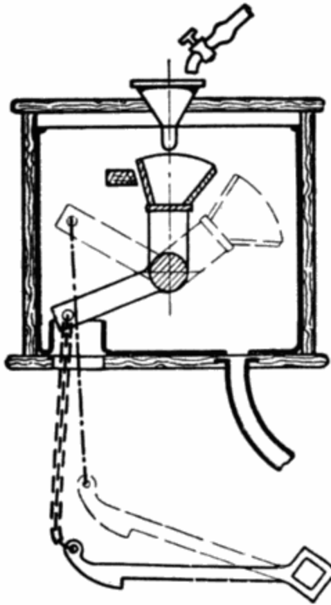
Abb. 11. Katarakt.
