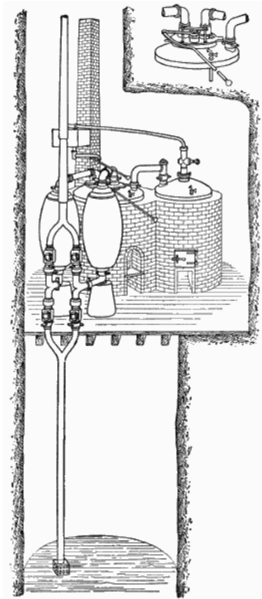
Abb. 7. Saverys Dampfpumpe.
