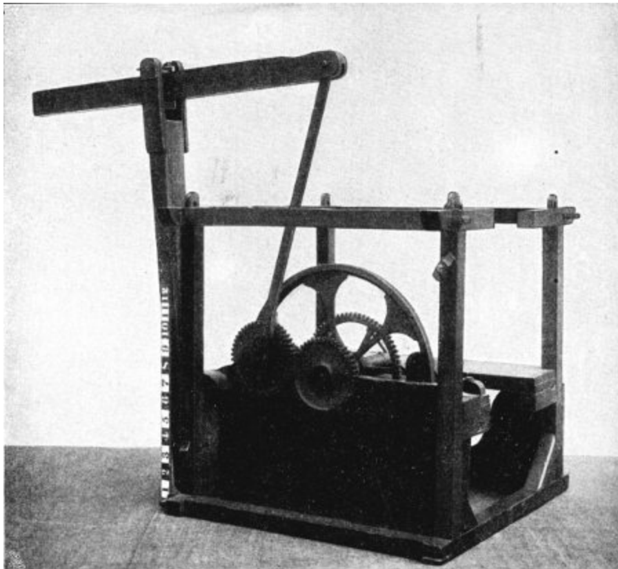
Abb. 18. Sonnen- und Planetenradgetriebe.
