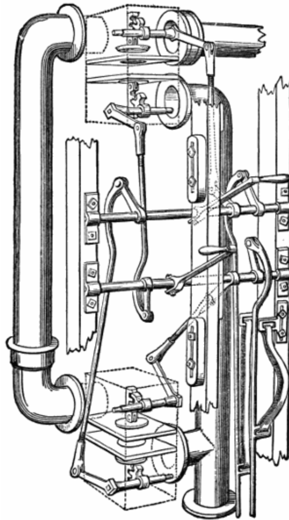
Abb. 16. Steuerung an den ersten doppelwirkenden Wattschen Maschinen.
