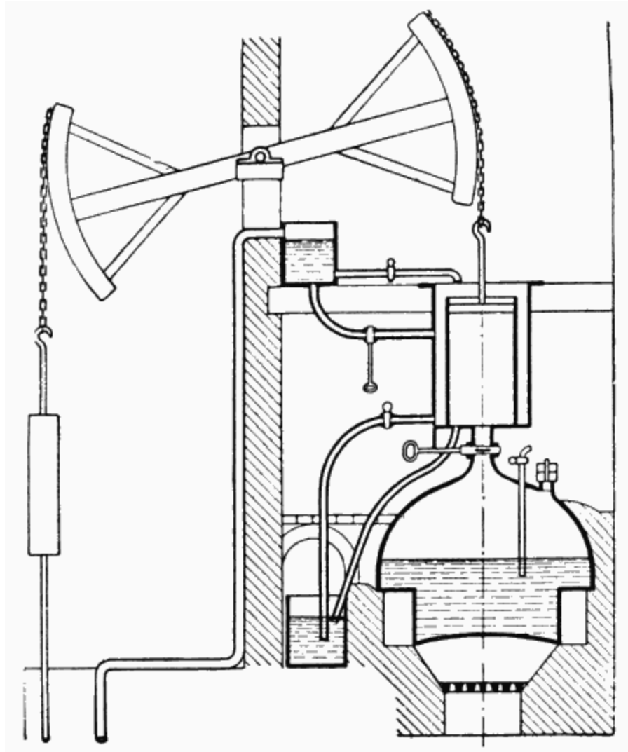
Abb. 9. Newcomenmaschine 1712.
