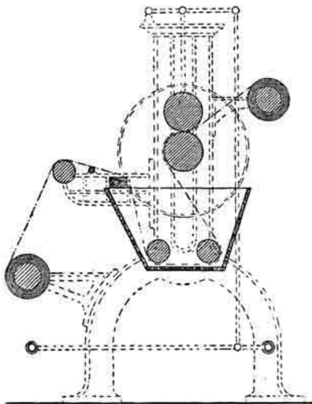
FIG. 25.—Padding Machine.
