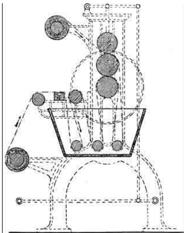
FIG. 26.—Padding Machine.
