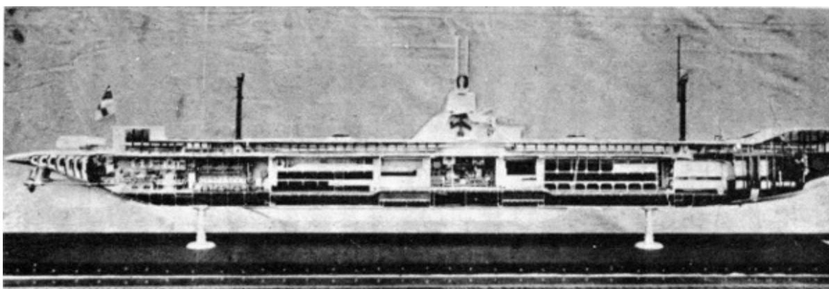
Innenansicht eines U-Bootes.
