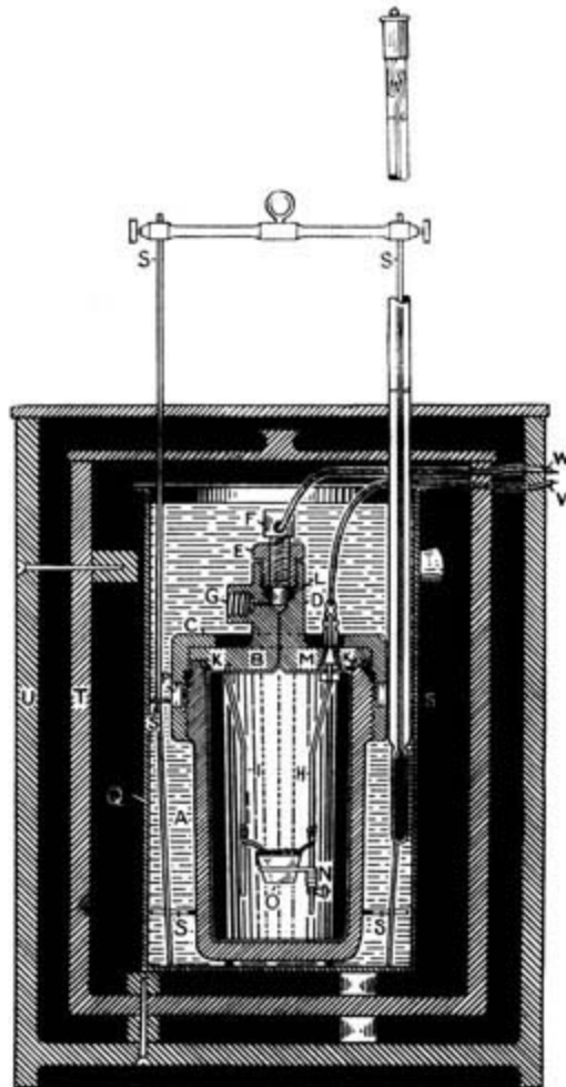
FIG. 55.—CALORIMETER.
