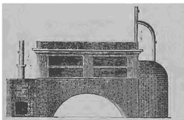
Nouveau système de Four, par M. Daudin-Langlois.--Élévation. Coupe du nouveau Four.
