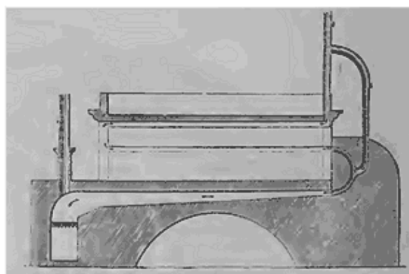
Nouveau système de Four, par M. Daudin-Langlois.--Élévation. Coupe du nouveau Four.
