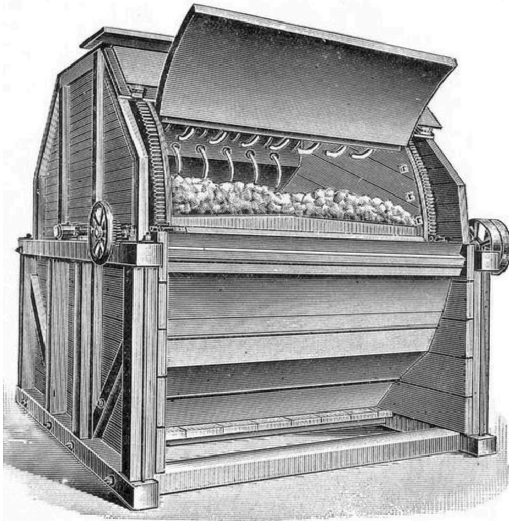
FIG. 12.—Delahunty's Dyeing Machine.
