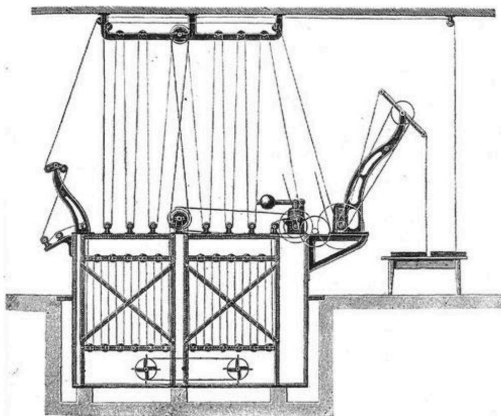
FIG. 23.—Indigo Dye-vat.
