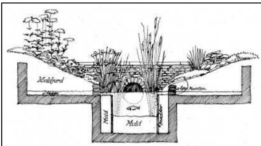
Fig. 8. Snit af „Grøften“ Fig. 7. Bredden foroven er ca. 4 Meter.
