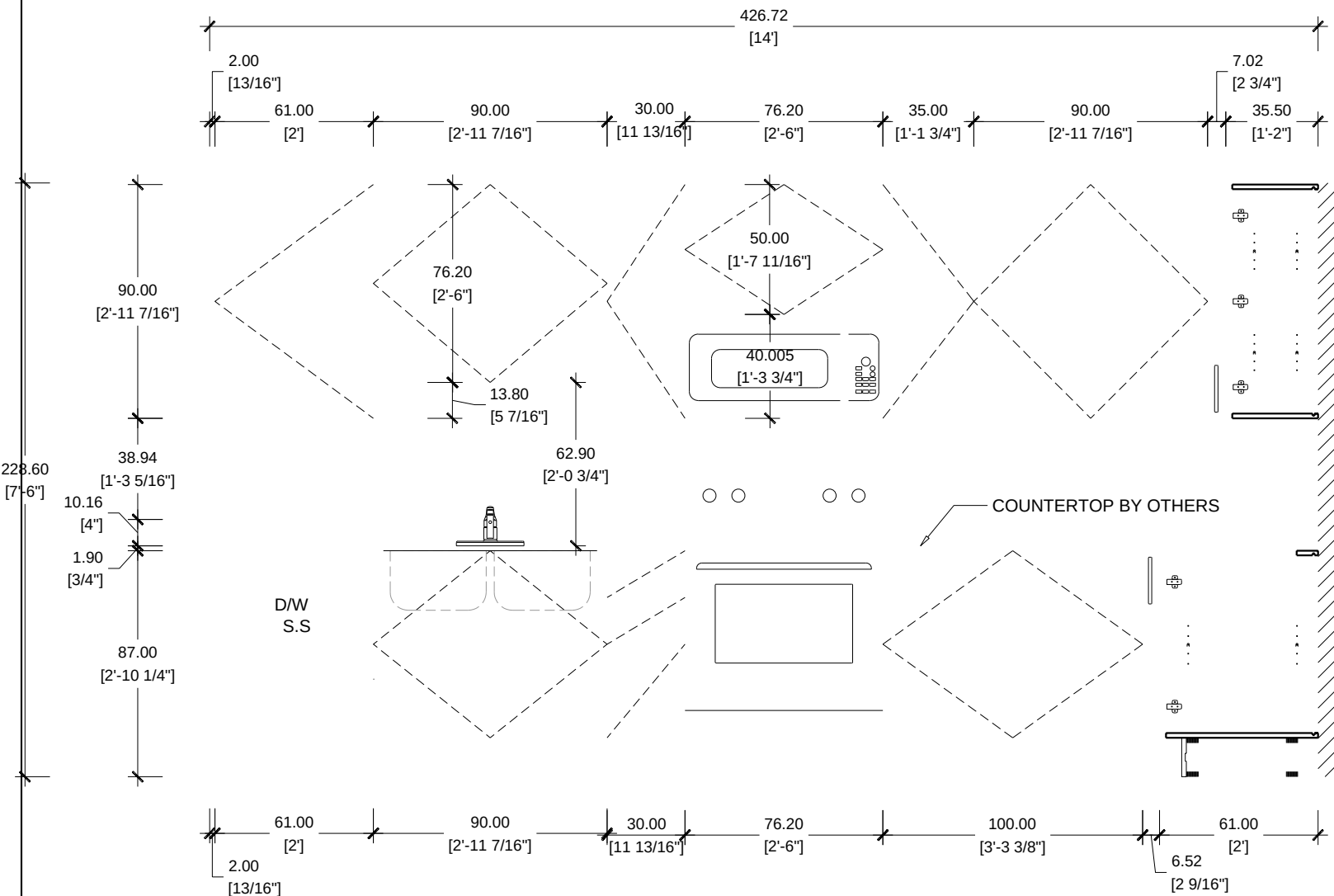
ELEVATION A
