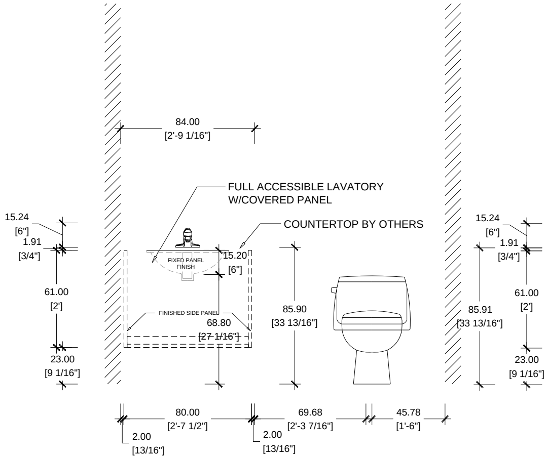
ELEVATION A CASA FAMILIA UNIT A2 FA / VANITY TYPE V2
