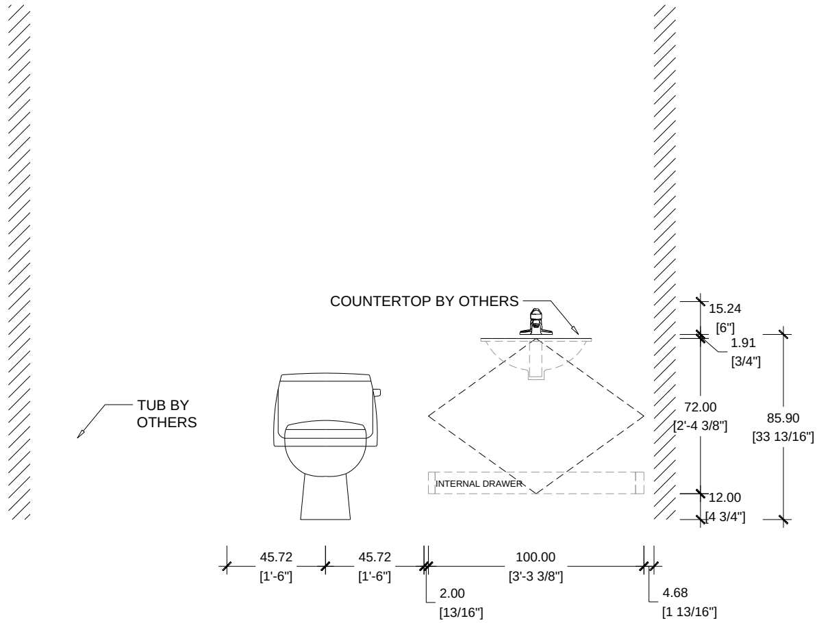
ELEVATION A CASA FAMILIA UNIT A3 / VANITY TYPE V3
