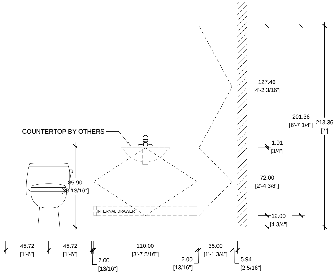
ELEVATION A CASA FAMILIA UNIT A1 / VANITY TYPE V1
