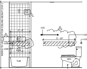
UNIT A-1 BATHROOM ELEV. SCALE: 1/2" = 1'-0"
