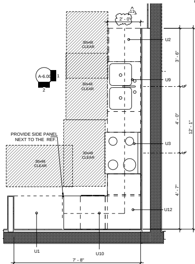
UNIT A-1 - KITCHEN SCALE: 1/2" = 1'-0"
