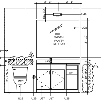
UNIT A-1 BATHROOM ELEV. SCALE: 1/2" = 1'-0"
