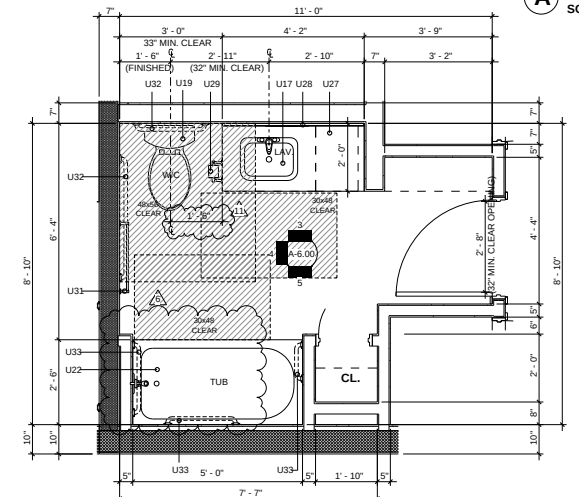
UNIT A-1 - BATHROOM SCALE: 1/2" = 1'-0"
