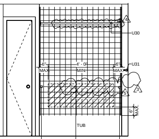
UNIT A-1 BATHROOM ELEV. SCALE: 1/2" = 1'-0"
