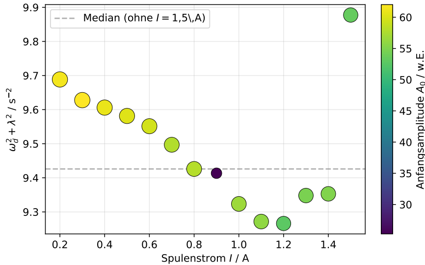
Abbildung 6: Implizites \omega_0^2 = \omega_d^2 + \lambda^2 aus jeder CASSY-Anpassung gegen den Spulenstrom I . Die Färbung der Punkte codiert die Anfangsamplitude A_0 ; die gestrichelte Linie ist der Median über alle Messungen mit I \leq 1,4 A.
