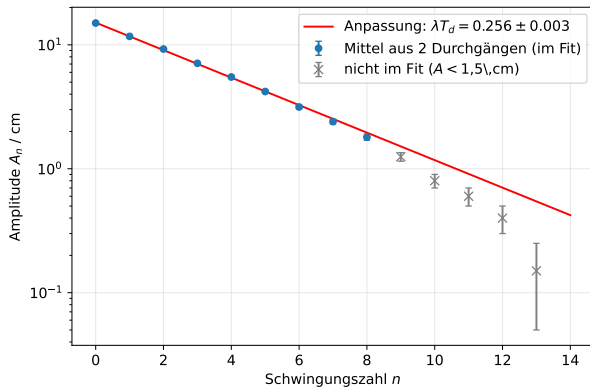
(a) Augen-Amplituden. Blau: A > 1,5 cm, im Fit enthalten. Grau: kleinere Amplituden, von der Geraden klar nach unten abweichend.
