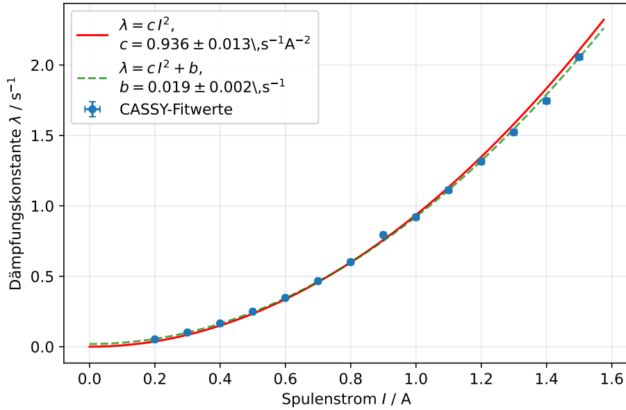
Abbildung 3: Dämpfungskonstante \lambda gegen Spulenstrom I . Rote Kurve: Anpassung \lambda = cI^2 . Grün gestrichelt: Anpassung mit zusätzlichem freien Achsenabschnitt.
