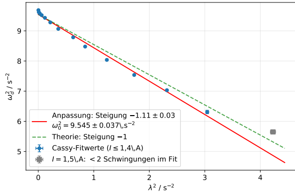
(a) Quadrate \omega_d^2 gegen \lambda^2 mit ungewichteter linearer Anpassung (rot) und theoretischer Steigung -1 (grün gestrichelt).
