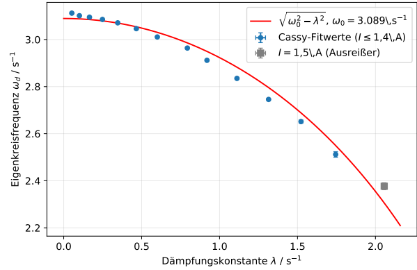
(b) Direktauftragung \omega_d gegen \lambda mit theoretischer Kurve \sqrt{\omega_0^2 - \lambda^2} ( \omega_0 = 3,089 \text{ s}^{-1} ).
