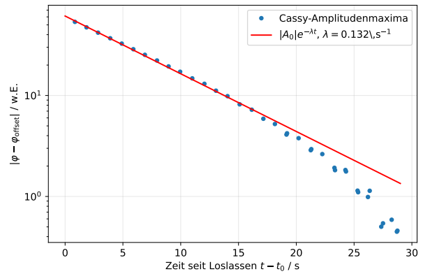
(b) Lokale Amplitudenmaxima des CASSY-Signals und Exponentialfunktion mit \lambda^{\text{CASSY}} .
