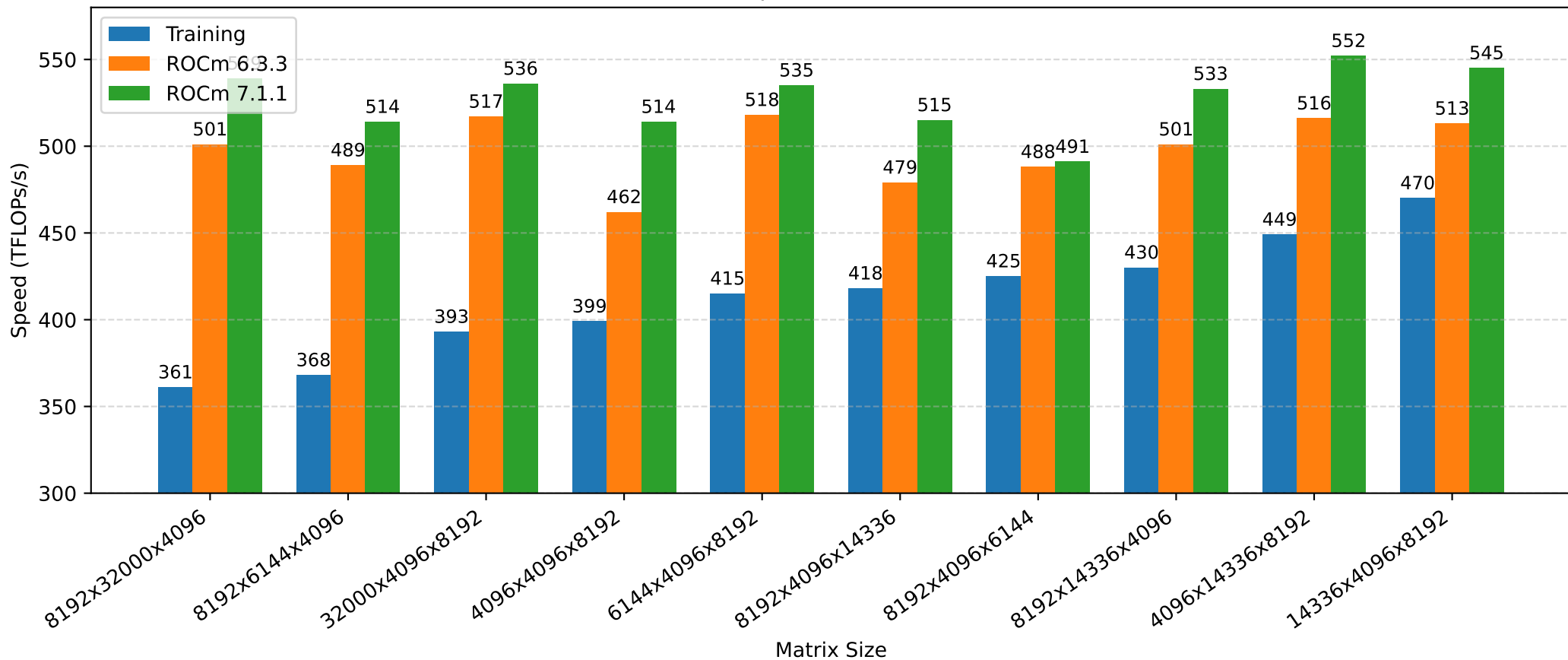
GEMM Speed (AMD MI300A)
