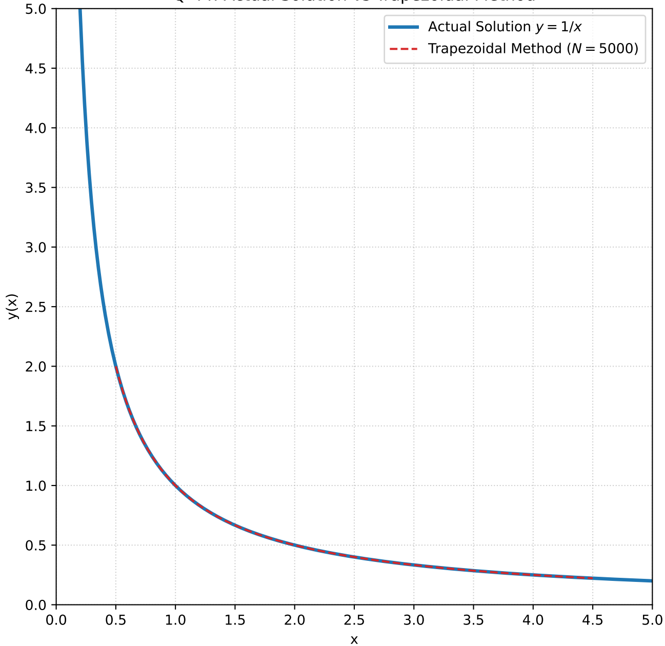
Q-44: Actual Solution vs Trapezoidal Method
