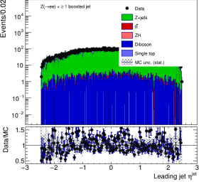
eta_jet_Z_jet_Zee_18_amcno.png
