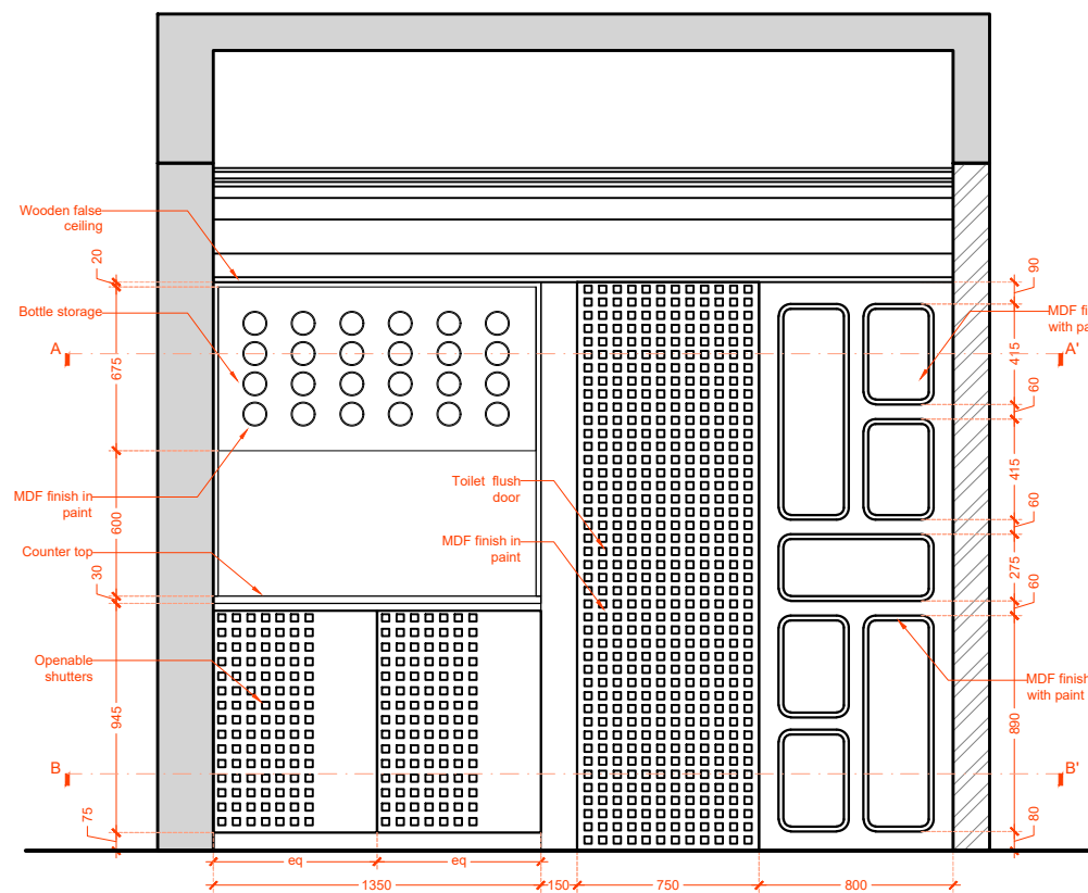
ELEVATION A1.01
