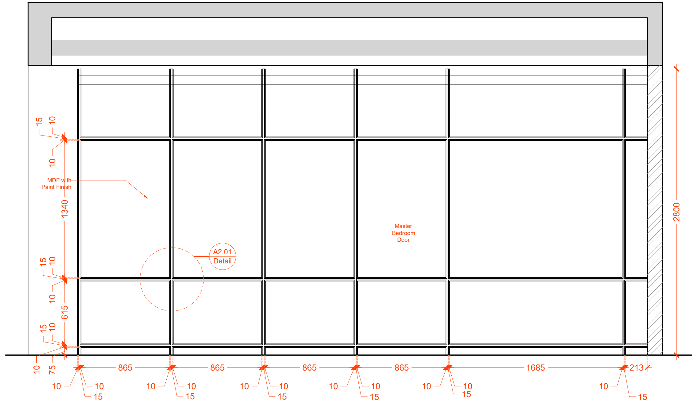
ELEVATION A2.01
