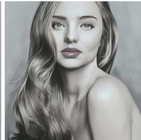
StyTR-2 CVPR'22
