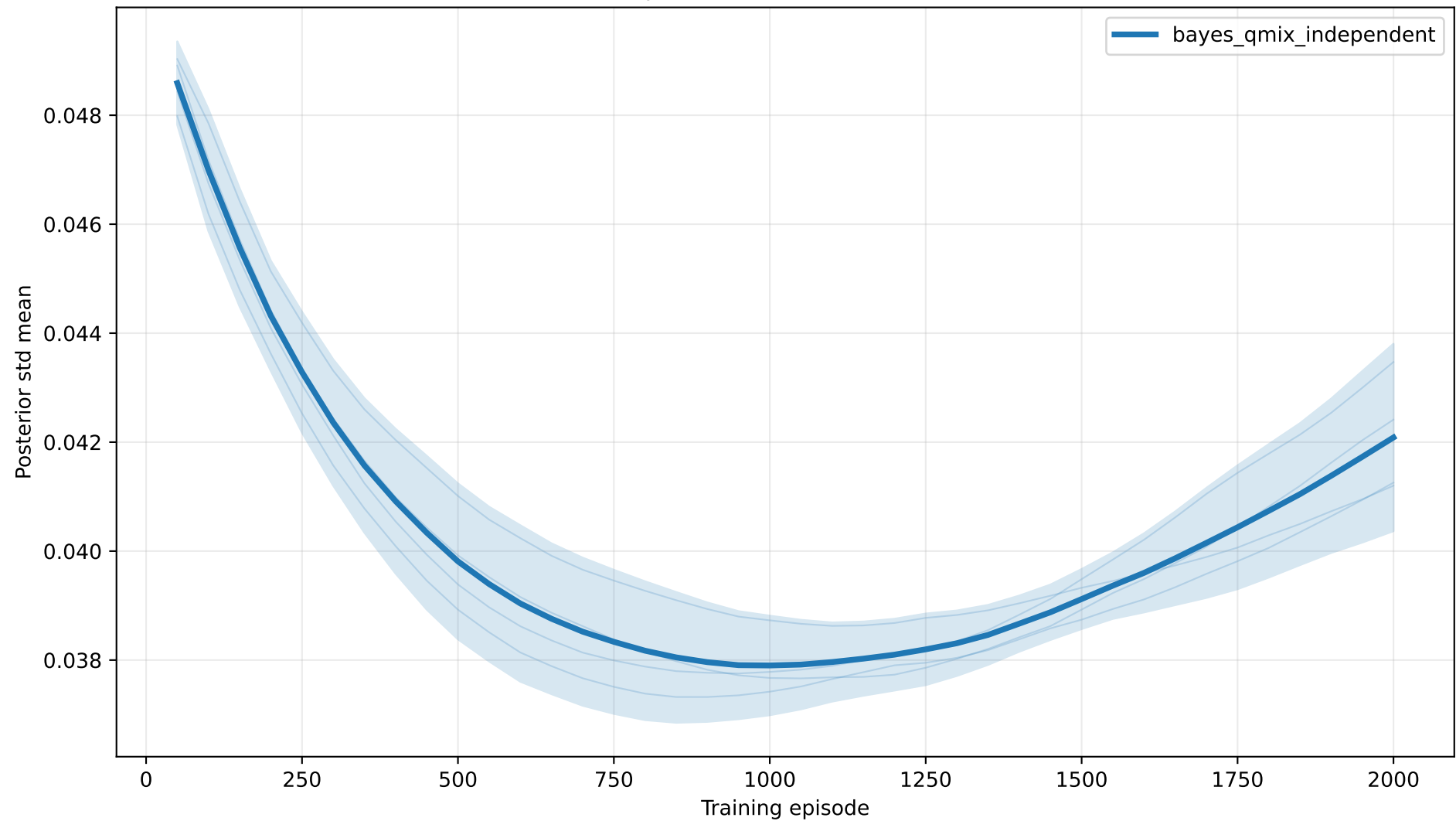
multi — pD=0.50 — Posterior std mean
