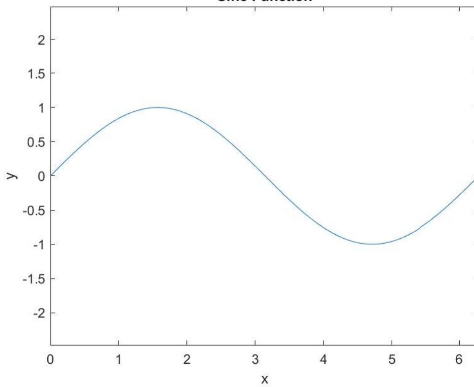
Sine Function
