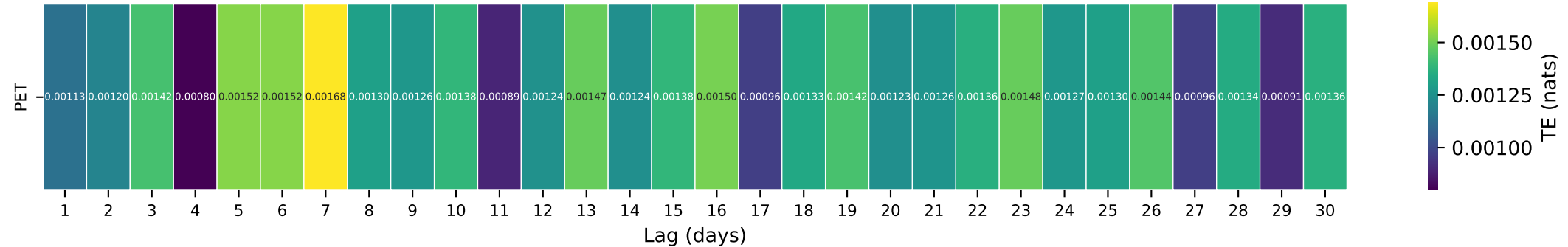
Gauge ID: 08050800 | Timber Ck nr Collinsville, TX | PET(t-\tau) \rightarrow Q(t)
