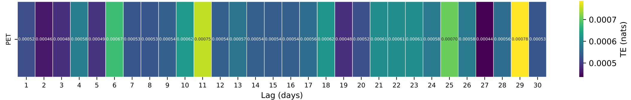
Gauge ID: 08070200 | E Fk San Jacinto Rv nr New Caney, TX | PET(t-\tau) \rightarrow Q(t)
