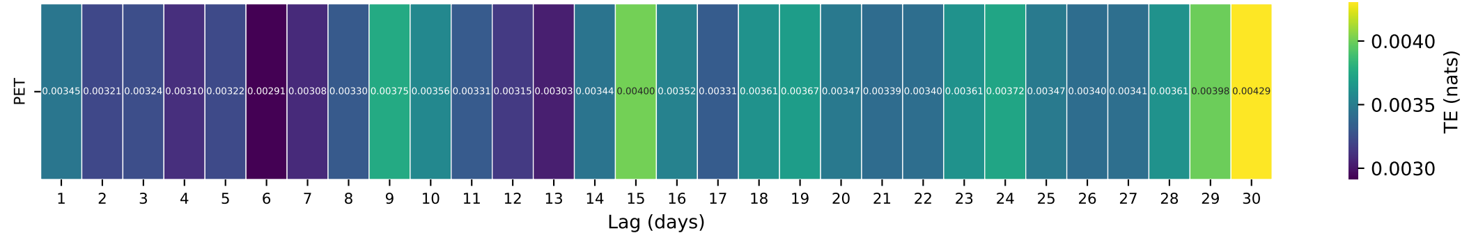
Gauge ID: 14308990 | COW CREEK ABV GALESVILLE RES, NR AZALEA, OR. | PET(t-\tau) \rightarrow Q(t)
