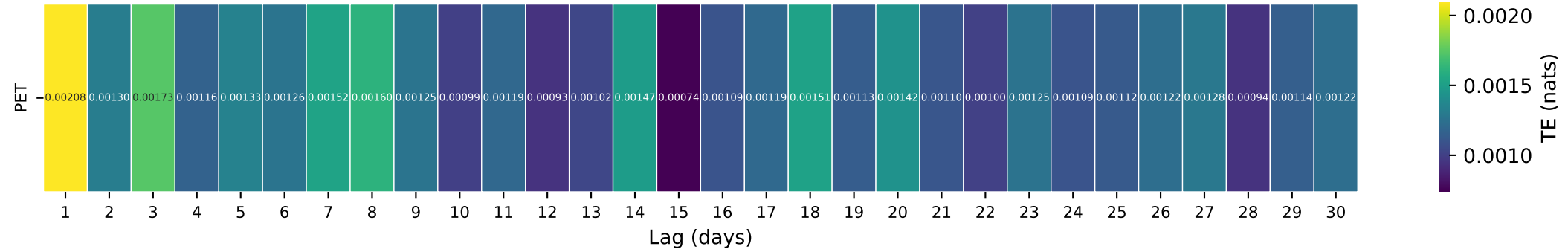
Gauge ID: 02246000 | NORTH FORK BLACK CREEK NR MIDDLEBURG, FLA. | PET(t-\tau) \rightarrow Q(t)
