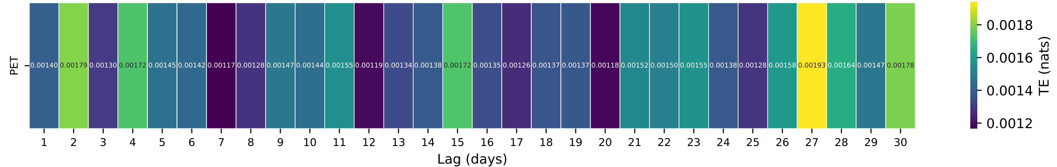
Gauge ID: 08164300 | Navidad Rv nr Hallettsville, TX | PET(t- \tau ) \rightarrow Q(t)
