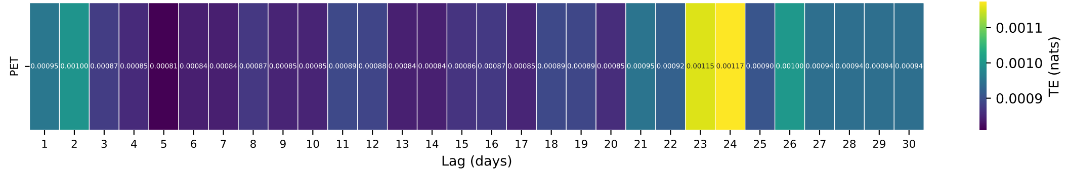
Gauge ID: 10259000 | ANDREAS C NR PALM SPRINGS CA | PET( t-\tau ) \rightarrow Q( t )
