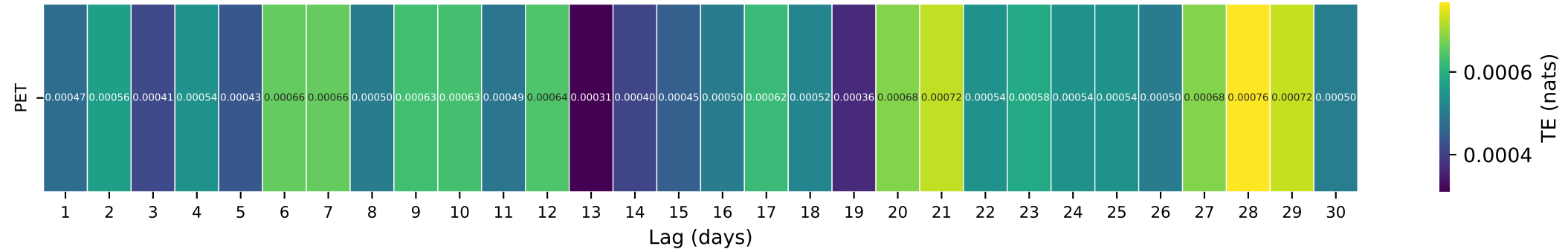
Gauge ID: 08190500 | W Nueces Rv nr Brackettville, TX | PET(t-\tau) \rightarrow Q(t)
