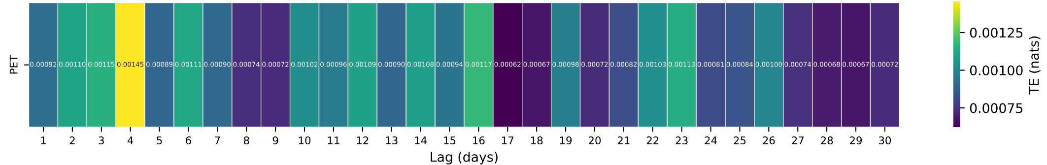
Gauge ID: 10343500 | SAGEHEN C NR TRUCKEE CA | PET(t- \tau ) \rightarrow Q(t)
