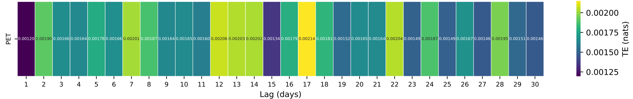
Gauge ID: 07180500 | CEDAR C NR CEDAR POINT, KS | PET(t-\tau) \rightarrow Q(t)
