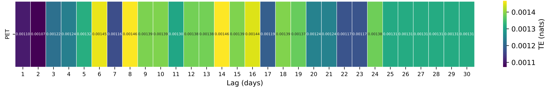
Gauge ID: 10263500 | BIG ROCK C NR VALYERMO CA | PET(t- \tau ) \rightarrow Q(t)
