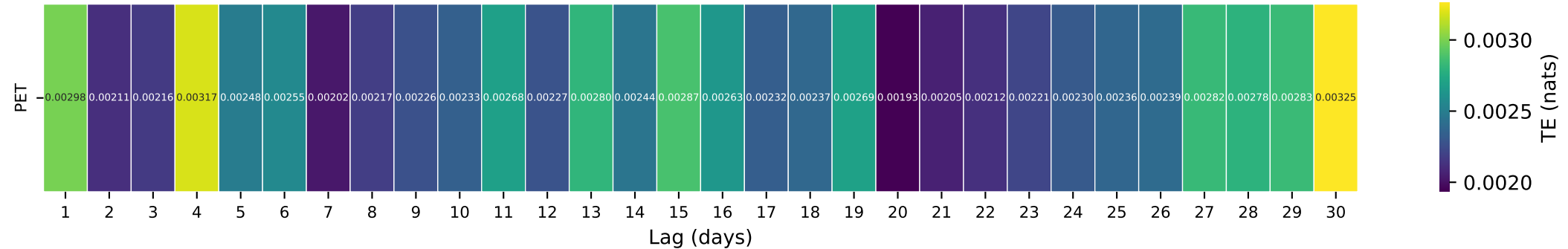
Gauge ID: 03291780 | INDIAN-KENTUCK CREEK NR CANAAN, IND. | PET(t-\tau) \rightarrow Q(t)
