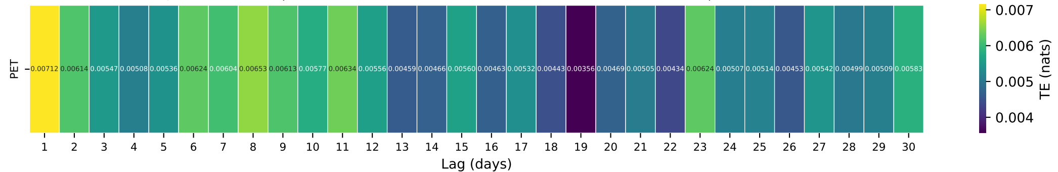
Gauge ID: 09210500 | FONTENELLE C NR HERSCHLER RANCH, NR FONTENELLE, WY | PET(t-\tau) \rightarrow Q(t)
