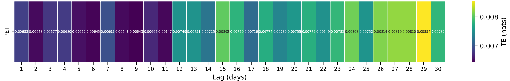
Gauge ID: 11478500 | VAN DUZEN R NR BRIDGEVILLE CA | PET(t-\tau) \rightarrow Q(t)
