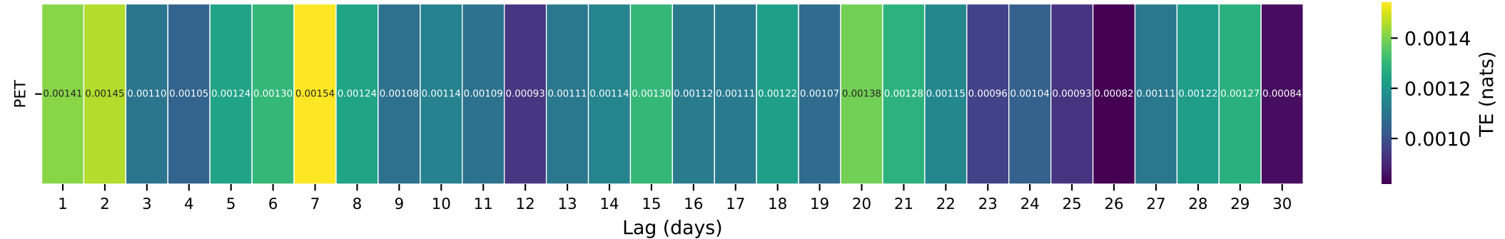
Gauge ID: 08109700 | Middle Yegua Ck nr Dime Box, TX | PET(t-\tau) \rightarrow Q(t)
