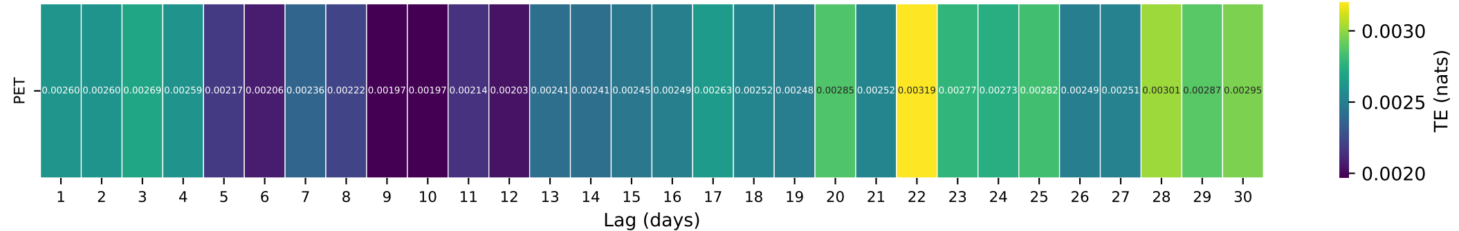
Gauge ID: 11148900 | NACIMIENTO R BL SAPAQUE C NR BRYSON CA | PET(t- \tau ) \rightarrow Q(t)
