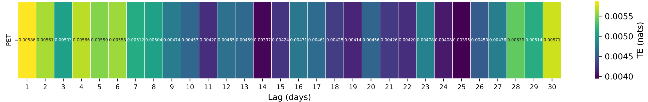
Gauge ID: 10396000 | DONNER UND BLITZEN RIVER NR FRENCHGLEN OR | PET(t-\tau) \rightarrow Q(t)
