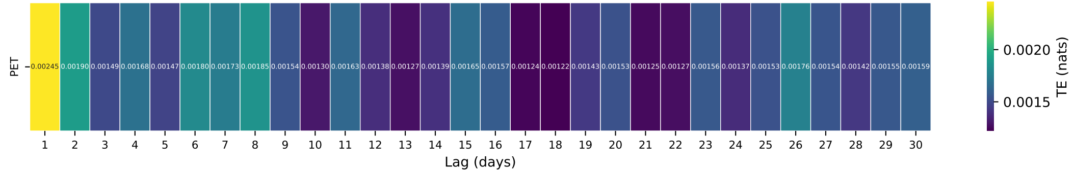
Gauge ID: 06332515 | BEAR DEN CREEK NR MANDAREE, ND | PET(t-\tau) \rightarrow Q(t)
