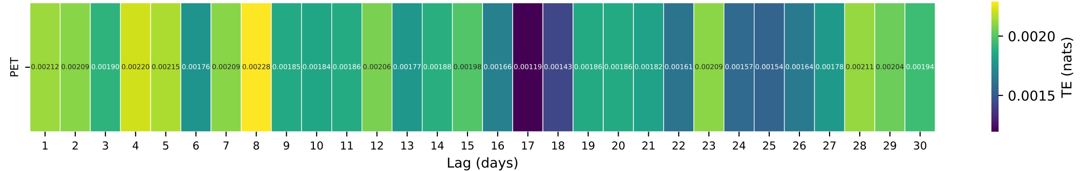
Gauge ID: 08013000 | CALCASIEU RIVER NR GLENMORA, LA | PET(t-\tau) \rightarrow Q(t)
