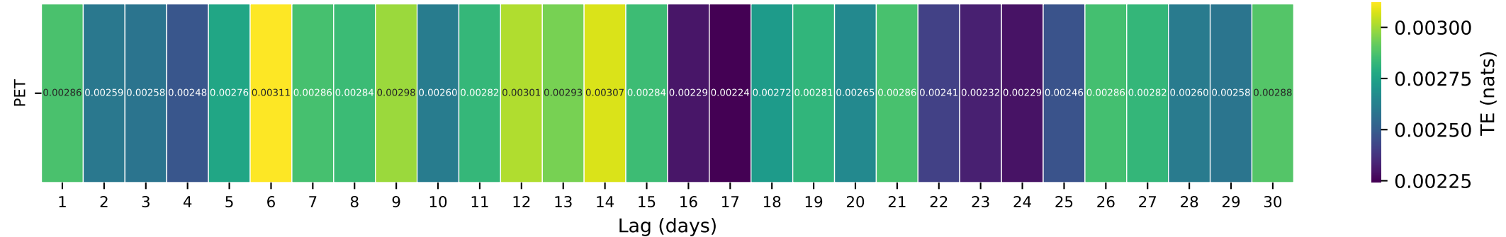
Gauge ID: 02430615 | MUD CREEK NR FAIRVIEW, MS | PET(t-\tau) \rightarrow Q(t)
