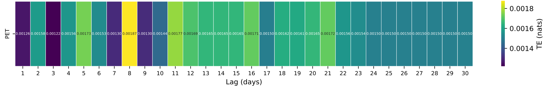
Gauge ID: 11098000 | ARROYO SECO NR PASADENA CA | PET(t- \tau ) \rightarrow Q(t)
