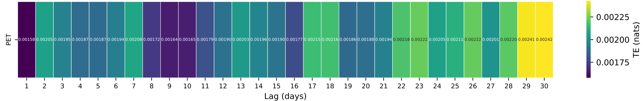
Gauge ID: 11124500 | SANTA CRUZ C NR SANTA YNEZ CA | PET(t-\tau) \rightarrow Q(t)
