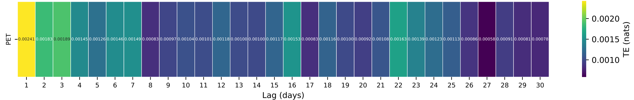
Gauge ID: 06479215 | BIG SIOUX RIVER NR FLORENCE SD | PET(t-\tau) \rightarrow Q(t)
