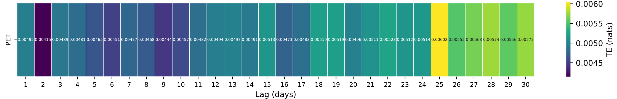
Gauge ID: 11481200 | LITTLE R NR TRINIDAD CA | PET(t- \tau ) \rightarrow Q(t)
