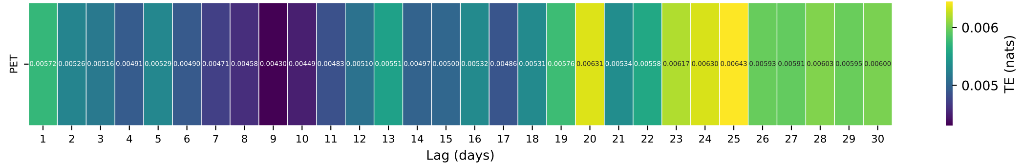
Gauge ID: 14158790 | SMITH R AB SMITH R RES NR BELKNAP SPRGS, OREG. | PET(t-\tau) \rightarrow Q(t)
