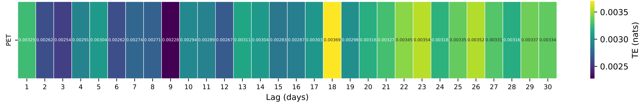
Gauge ID: 11162500 | PESCADERO C NR PESCADERO CA | PET(t- \tau ) \rightarrow Q(t)
