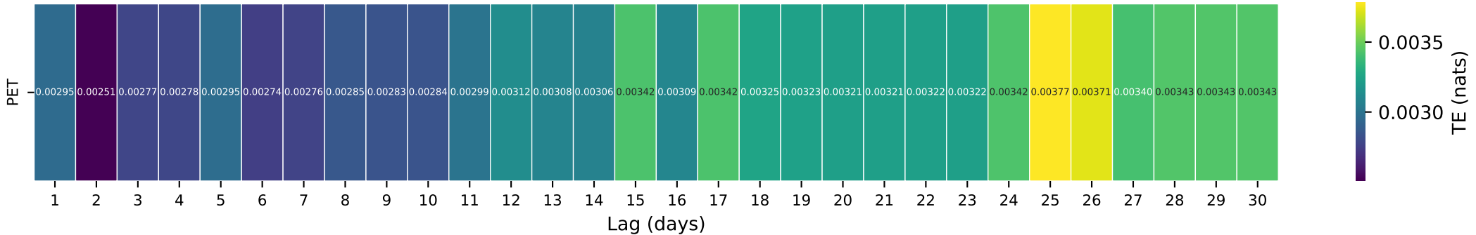
Gauge ID: 11473900 | MF EEL R NR DOS RIOS CA | PET(t- \tau ) \rightarrow Q(t)
