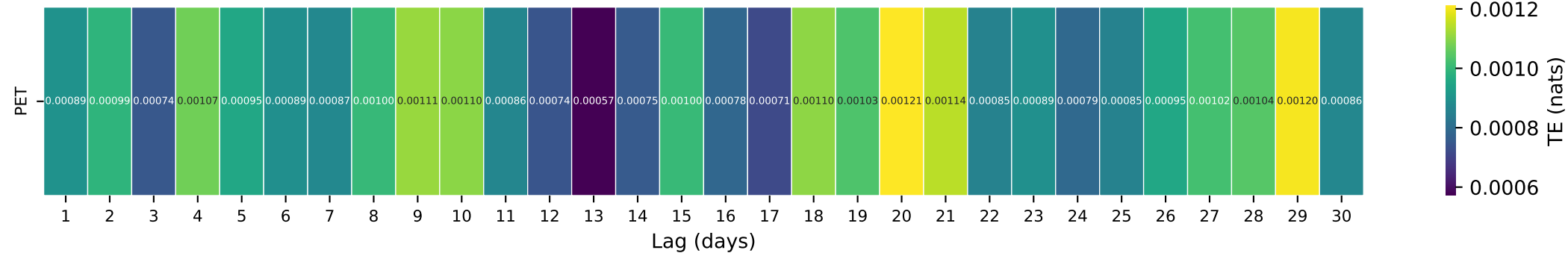
Gauge ID: 08190000 | Nueces Rv at Laguna, TX | PET(t-\tau) \rightarrow Q(t)
