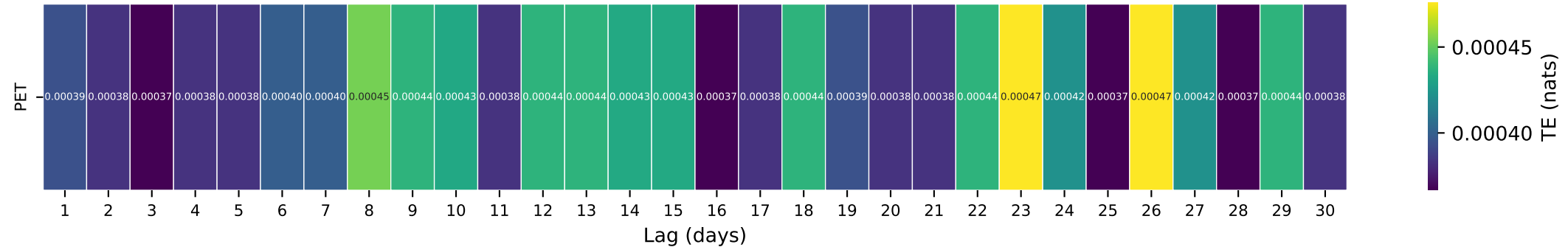
Gauge ID: 08082700 | Millers Ck nr Munday, TX | PET(t-\tau) \rightarrow Q(t)
