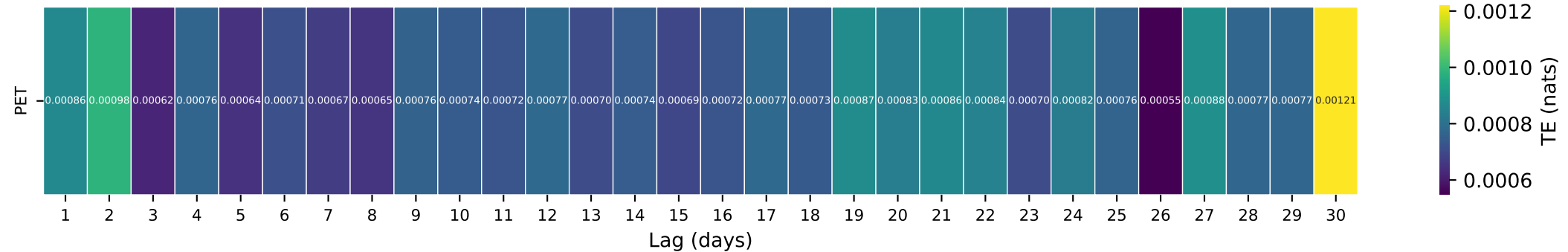
Gauge ID: 08175000 | Sandies Ck nr Westhoff, TX | PET(t-\tau) \rightarrow Q(t)
