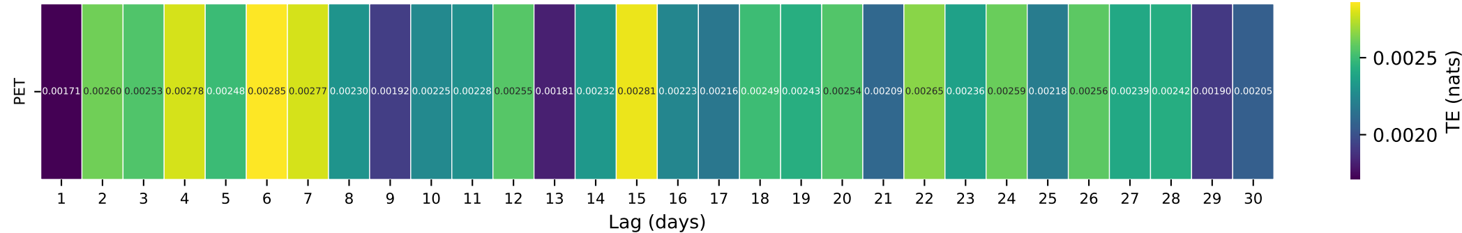
Gauge ID: 06888500 | MILL C NR PAXICO, KS | PET(t-τ) → Q(t)
