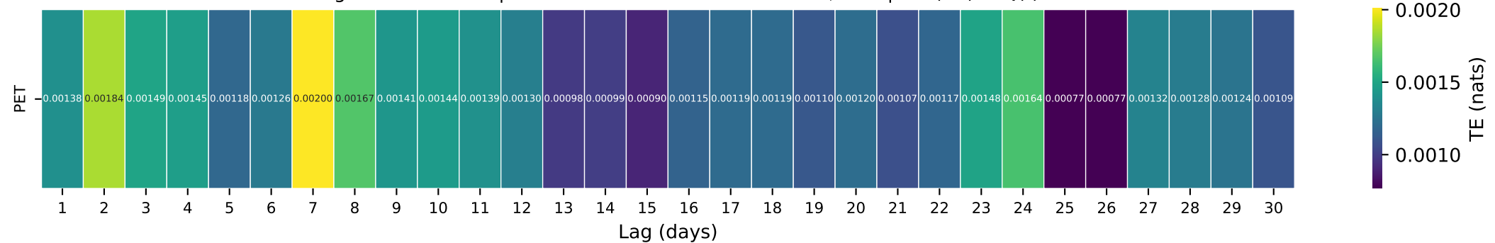
Gauge ID: 02231000 | ST. MARYS RIVER NR MACCLENNY, FLA. | PET(t-\tau) \rightarrow Q(t)
