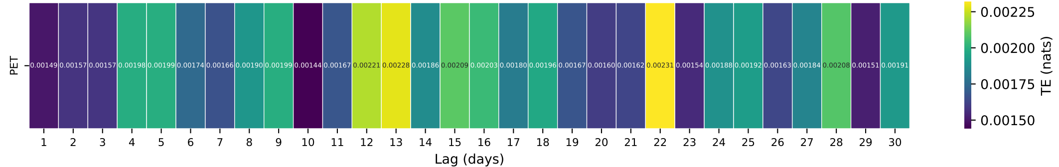
Gauge ID: 07151500 | CHIKASKIA R NR CORBIN, KS | PET(t-\tau) \rightarrow Q(t)
