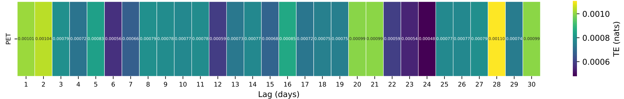
Gauge ID: 08165300 | N Fk Guadalupe Rv nr Hunt, TX | PET(t-\tau) \rightarrow Q(t)
