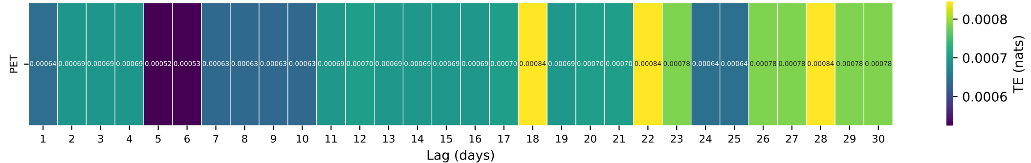
Gauge ID: 11151300 | SAN LORENZO C BL BITTERWATER C NR KING CITY CA | PET(t-\tau) \rightarrow Q(t)
