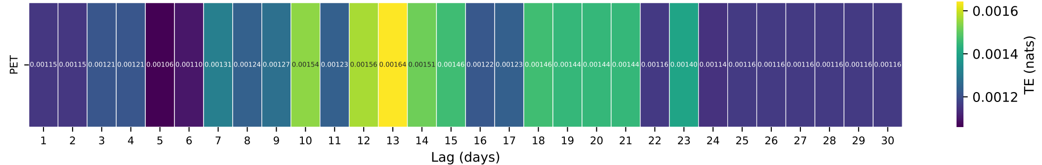
Gauge ID: 11274630 | DEL PUERTO C NR PATTERSON CA | PET(t-\tau) \rightarrow Q(t)
