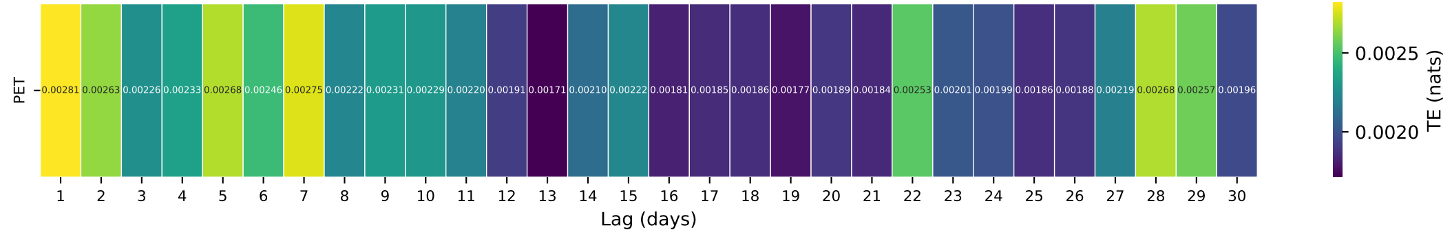
Gauge ID: 10329500 | MARTIN C NR PARADISE VALLEY, NV | PET(t-\tau) \rightarrow Q(t)
