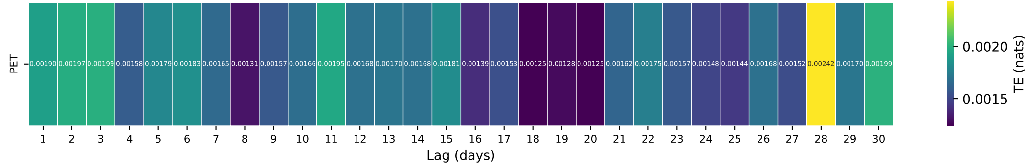
Gauge ID: 08164000 | Lavaca Rv nr Edna, TX | PET(t-\tau) \rightarrow Q(t)
