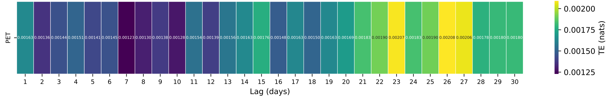
Gauge ID: 11381500 | MILL C NR LOS MOLINOS CA | PET(t- \tau ) \rightarrow Q(t)
