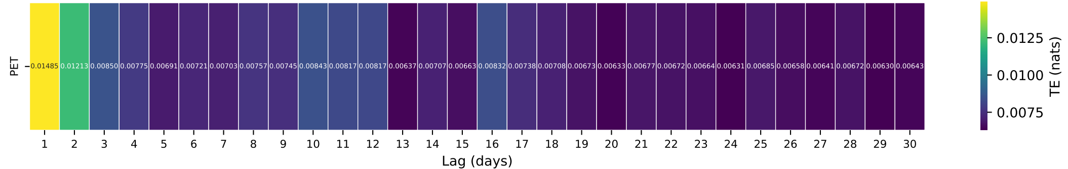
Gauge ID: 13011900 | BUFFALO FORK AB LAVA CREEK NR MORAN WY | PET(t-\tau) \rightarrow Q(t)
