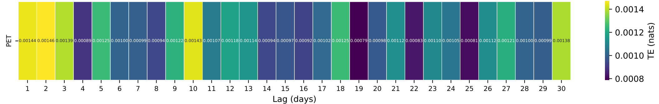
Gauge ID: 06352000 | CEDAR CREEK NR HAYNES, ND | PET(t-\tau) \rightarrow Q(t)
