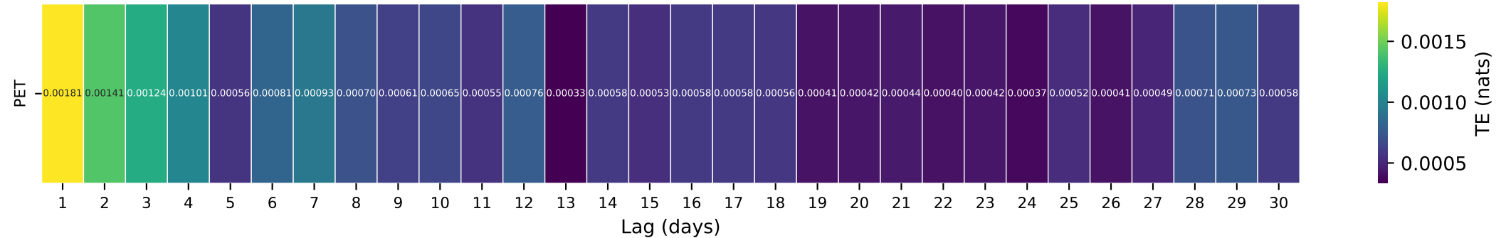
Gauge ID: 02327100 | SOPCHOPPY RIVER NR SOPCHOPPY, FLA. | PET(t-\tau) \rightarrow Q(t)
