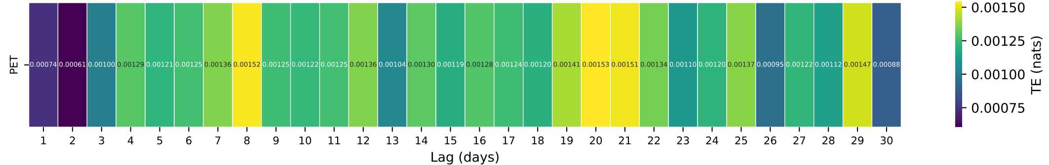
Gauge ID: 06910800 | MARAIS DES CYGNES R NR READING, KS | PET(t-\tau) \rightarrow Q(t)
