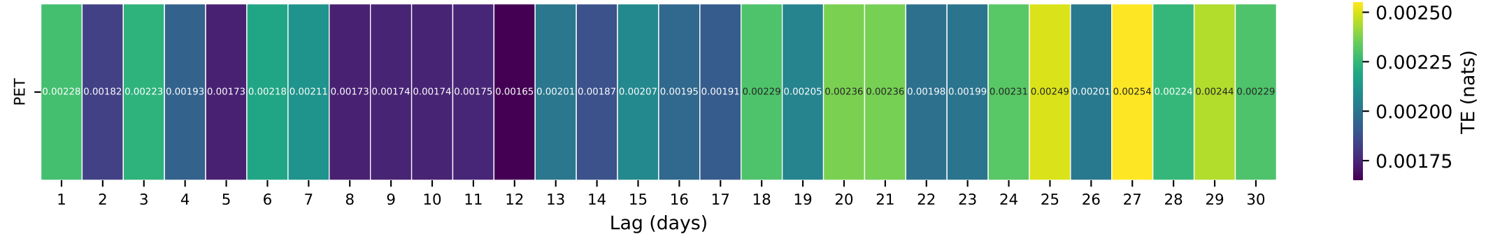
Gauge ID: 02430085 | RED BUD CREEK NR MOORES MILL, MS | PET(t-\tau) \rightarrow Q(t)
