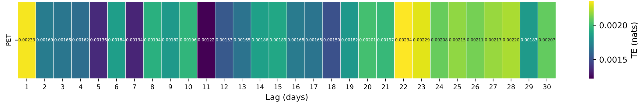
Gauge ID: 02472500 | BOUIE CREEK NR HATTIESBURG, MS | PET(t-\tau) \rightarrow Q(t)
