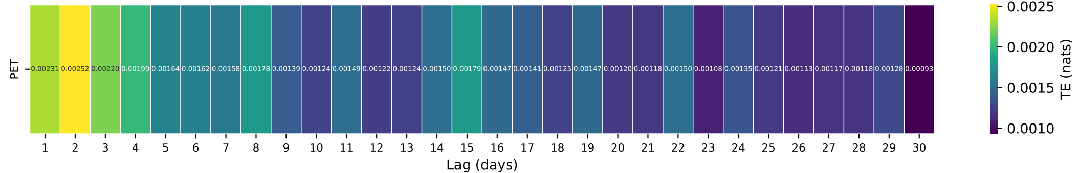
Gauge ID: 05057200 | BALDHILL CREEK NR DAZEY, ND | PET(t-\tau) \rightarrow Q(t)
