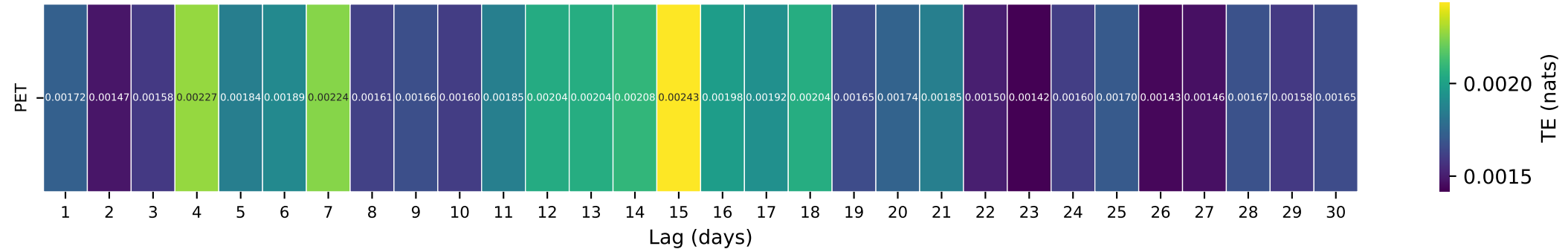
Gauge ID: 06889500 | SOLDIER C NR TOPEKA, KS | PET(t-\tau) \rightarrow Q(t)
