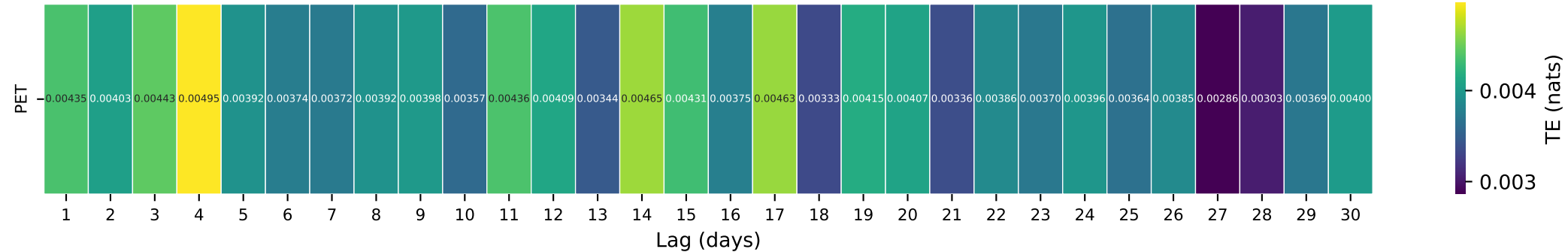
Gauge ID: 06814000 | TURKEY C NR SENECA, KS | PET(t-\tau) \rightarrow Q(t)
