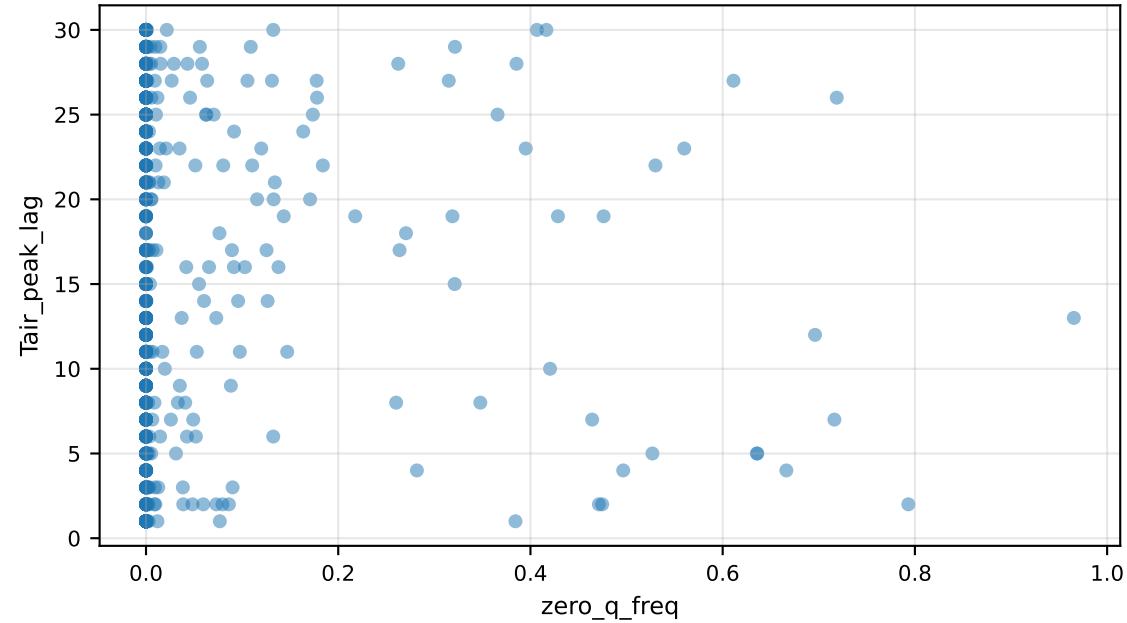
Tair_peak_lag vs zero_q_freq
