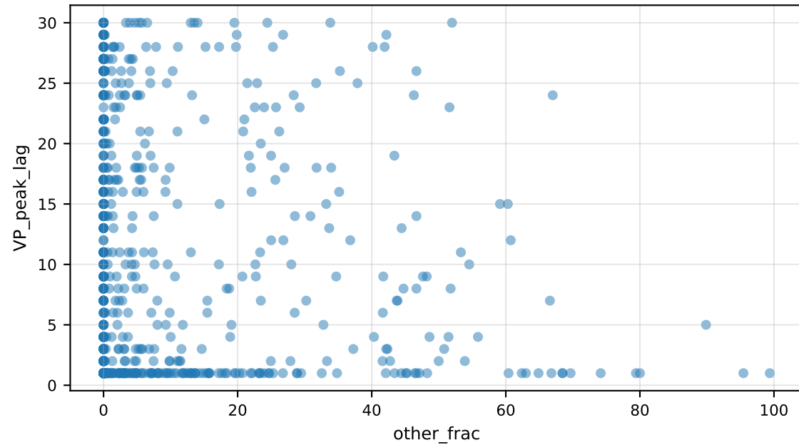
VP_peak_lag vs other_frac
