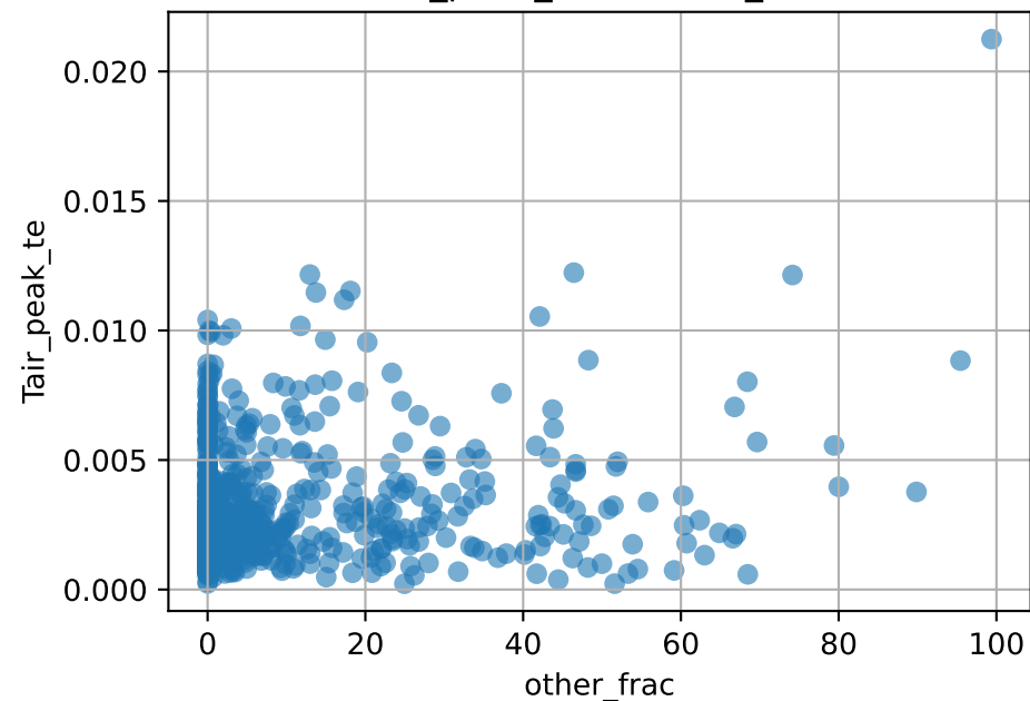
Tair_peak_te vs other_frac
