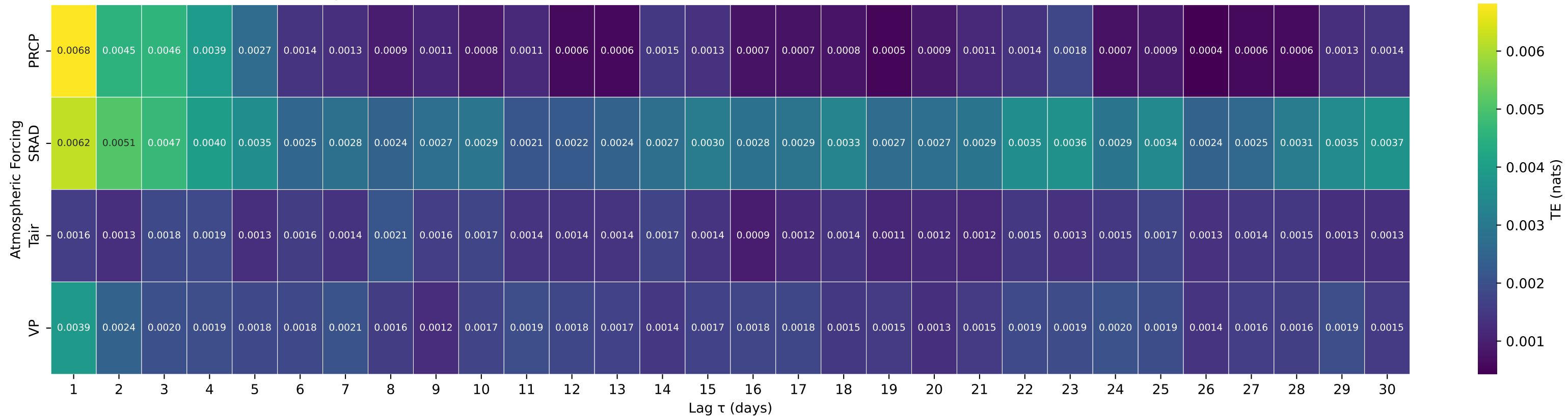
Shuffle-Test Significant TE to Streamflow — Basin 11148900 (HUC 18) — NACIMIENTO R BL SAPAQUE C NR BRYSON CA
