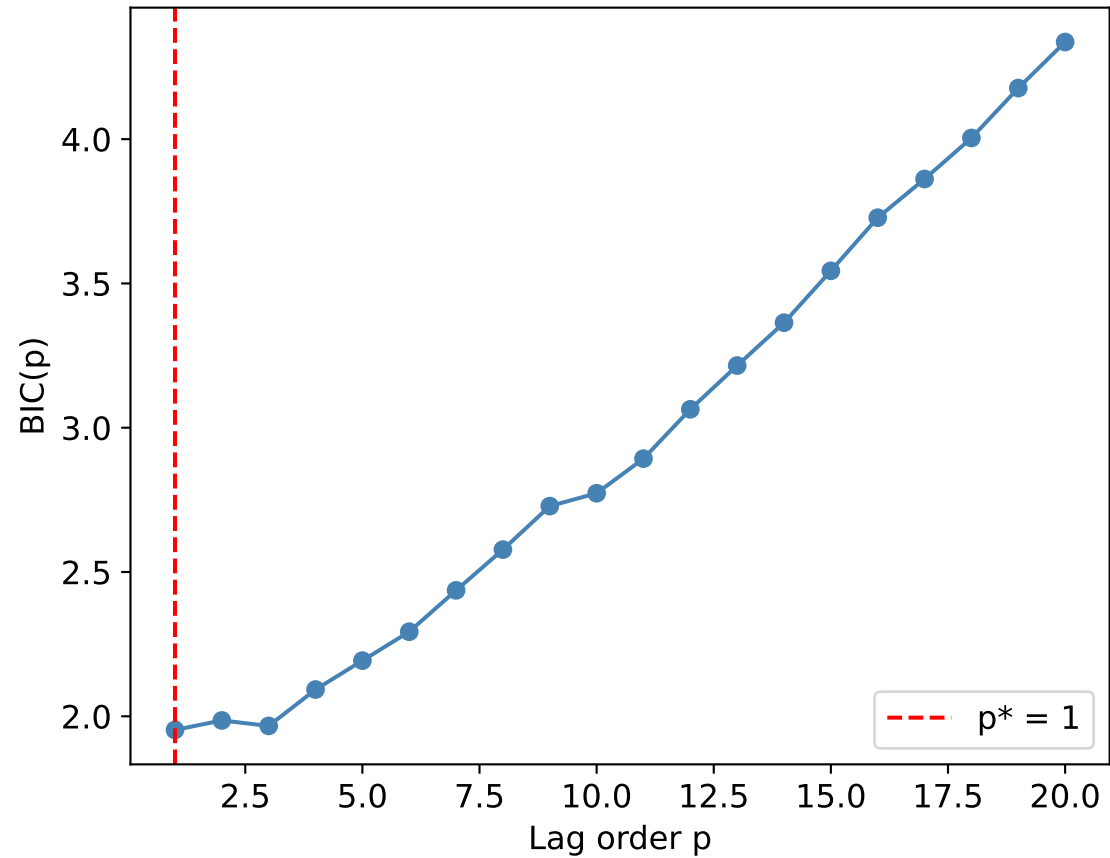
BIC
