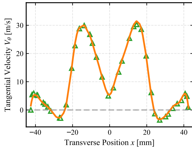
(d) Station z = 60 mm (Downstream Swirl Decay)
