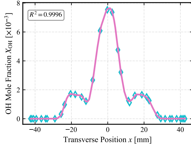
(d) Station z = 25 mm (Peak Radical Zone)
