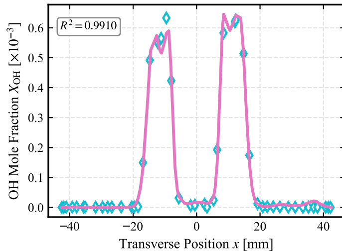
(d) Station z = 25 mm (Peak Radical Zone)
