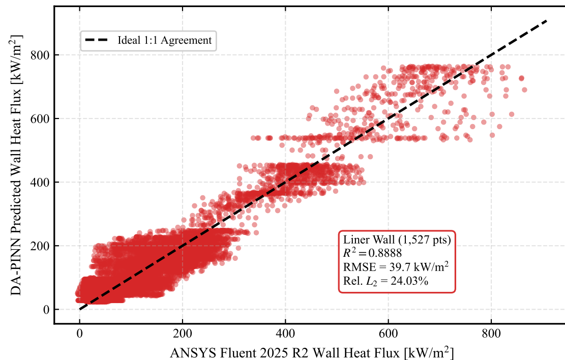
(d) Liner Wall Heat Flux Parity Scatter
