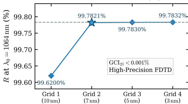
(d) Metasurface Reflectance R(\lambda_0)
