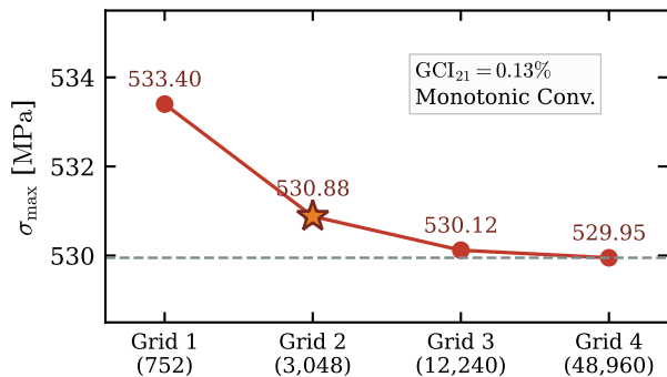
(a) Maximum Von Mises Stress \sigma_{\max}
