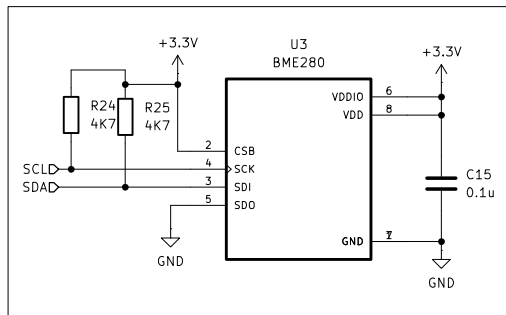
BME280
