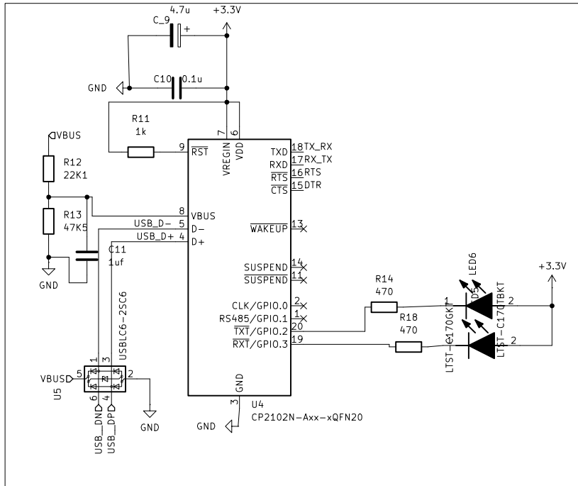
USB MODULE
