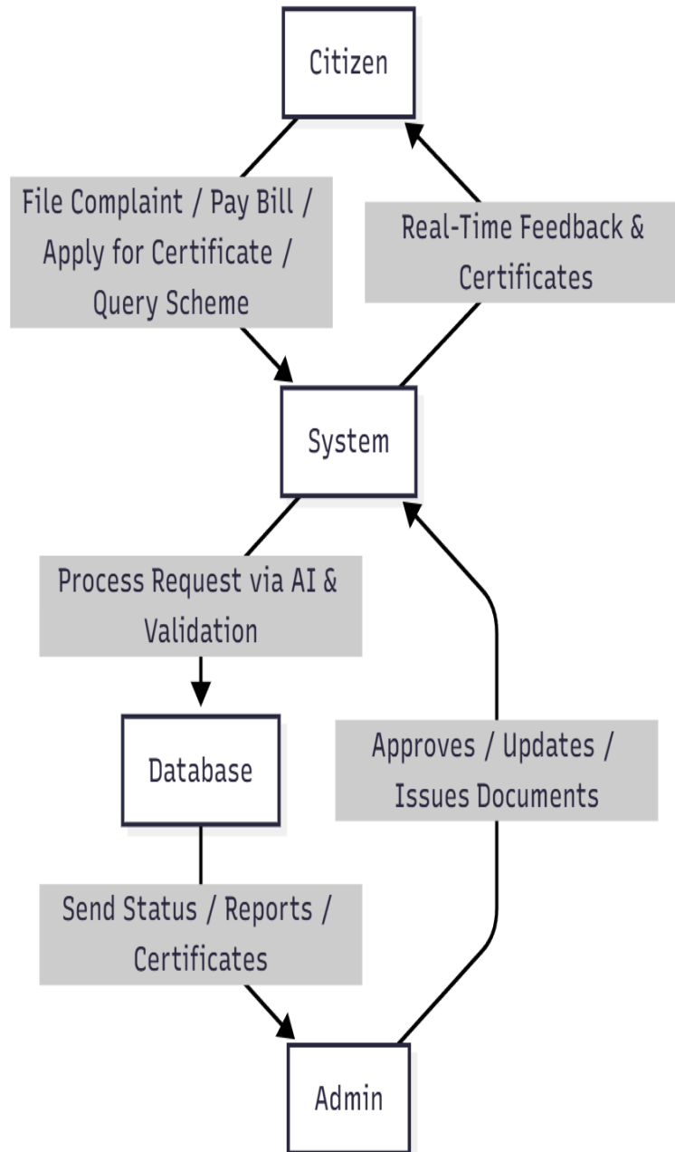
(Dfd 0)
