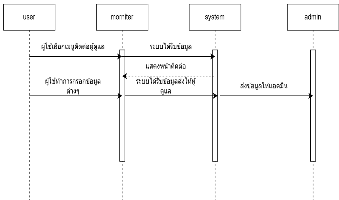
รูปที่ 3.5 แผนภาพแสดงลำดับการทำงาน ติดต่อผู้ดูแล
