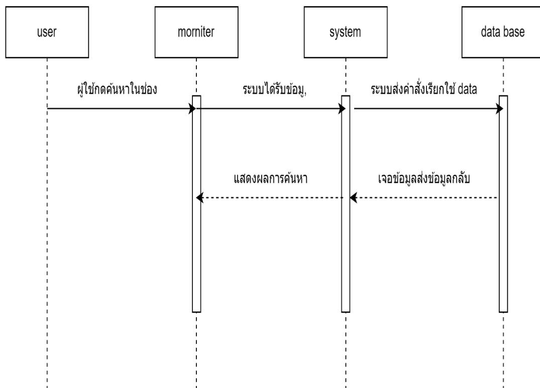
รูปที่ 3.10 แผนภาพแสดงลำดับการทำงาน ค้นหา
