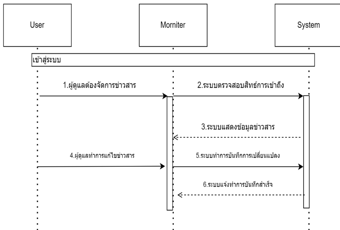
รูปที่ 3.9 แผนภาพแสดงลำดับการทำงาน จัดการข่าวสาร
