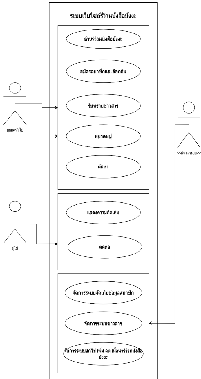
รูปที่ 3.1 แผนภาพแสดง Use Case Diagram
