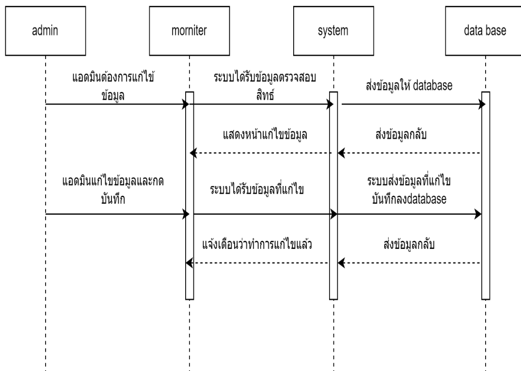
รูปที่ 3.8 แผนภาพแสดงลำดับการทำงาน จัดการระบบกำหนดข้อมูลแก้ไข
