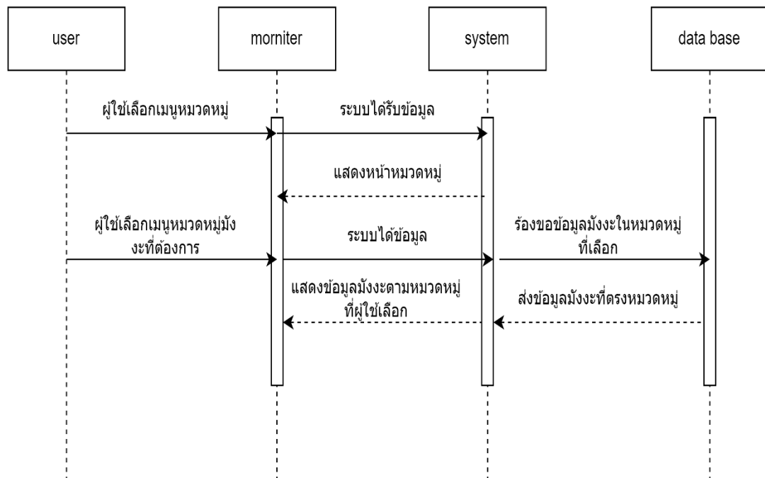
รูปที่ 3.11 แผนภาพแสดงลำดับการทำงาน หมวดหมู่
