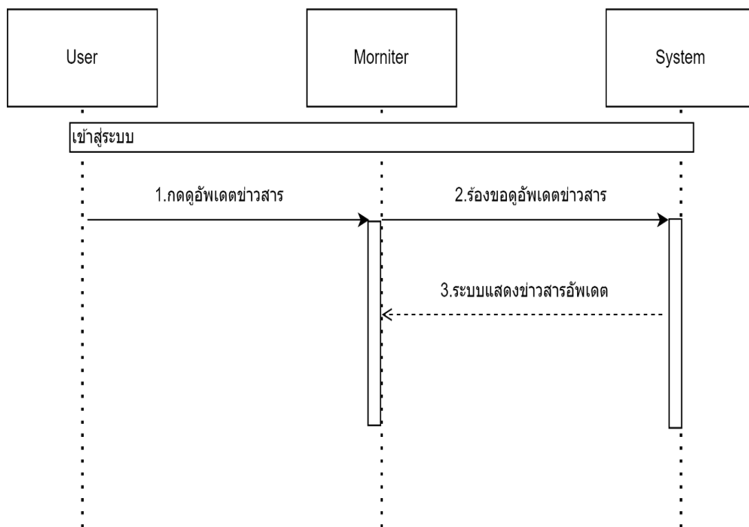
รูปที่ 3.4 แผนภาพแสดงลำดับการทำงาน รับข่าวสาร
