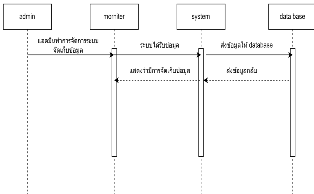
รูปที่ 3.6 แผนภาพแสดงลำดับการทำงาน จัดการระบบเก็บข้อมูลสมาชิก
