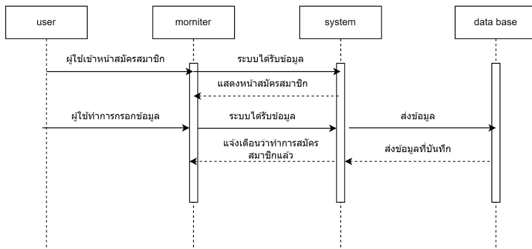
รูปที่ 3.2 แผนภาพแสดงลำดับการทำงานของระบบ การสมัครสมาชิก
