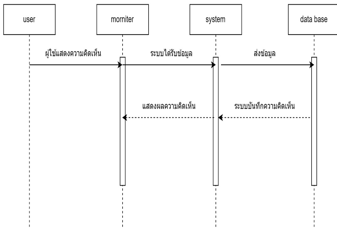
รูปที่ 3.7 แผนภาพแสดงลำดับการทำงาน แสดงความคิดเห็น
