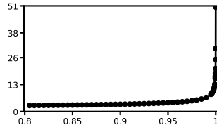
glove25
