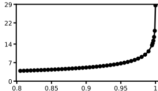
coco_i2i
