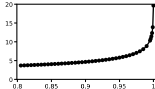
mnist
