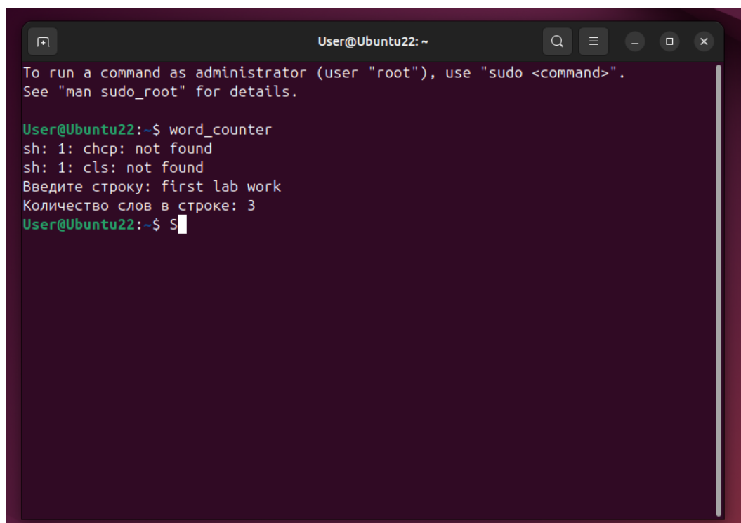
Рисунок 9 – запуск deb пакета
