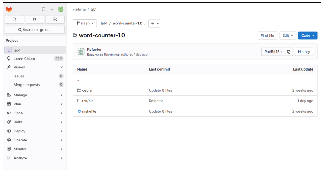
Рисунок 6 – Репозиторий Gitlab
