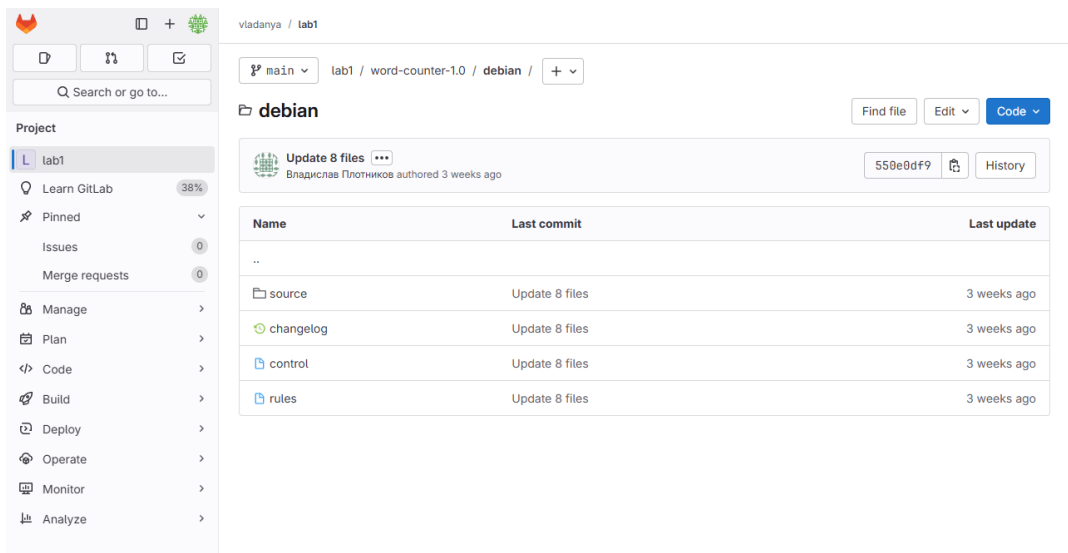
Рисунок 7 – Репозиторий Gitlab(debian)
