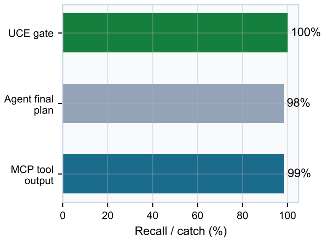
(d) Evidence → plan → enforcement
