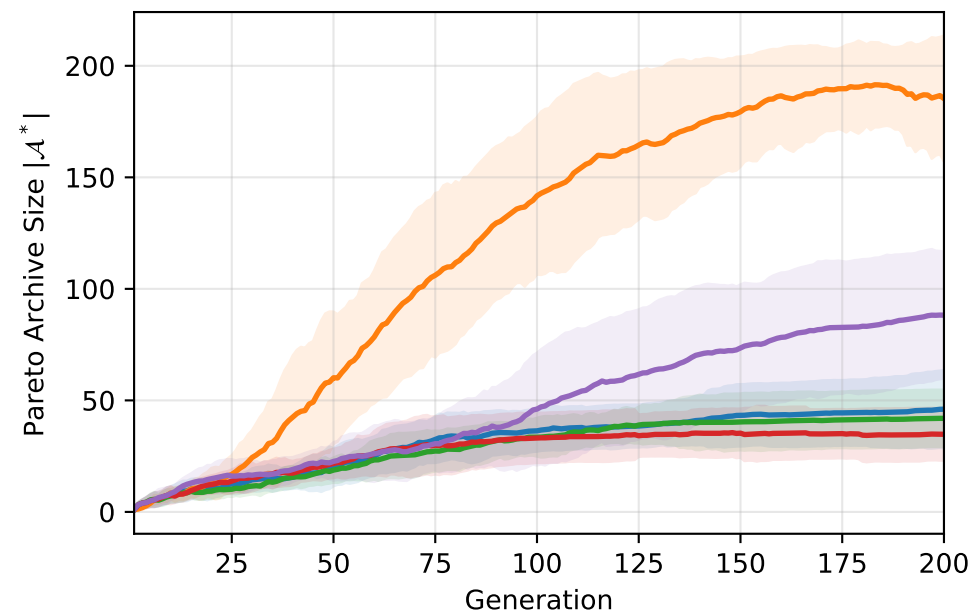
eil51
