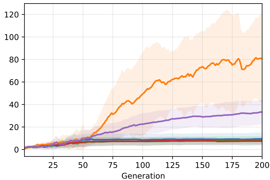
kroA100
