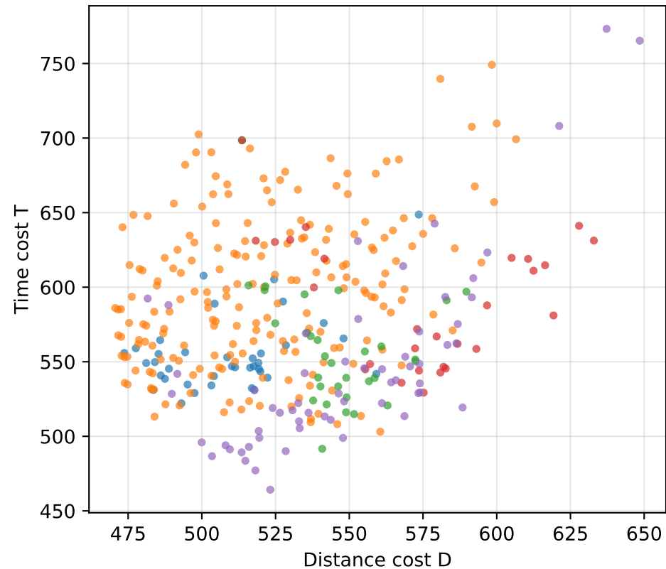
eil51
