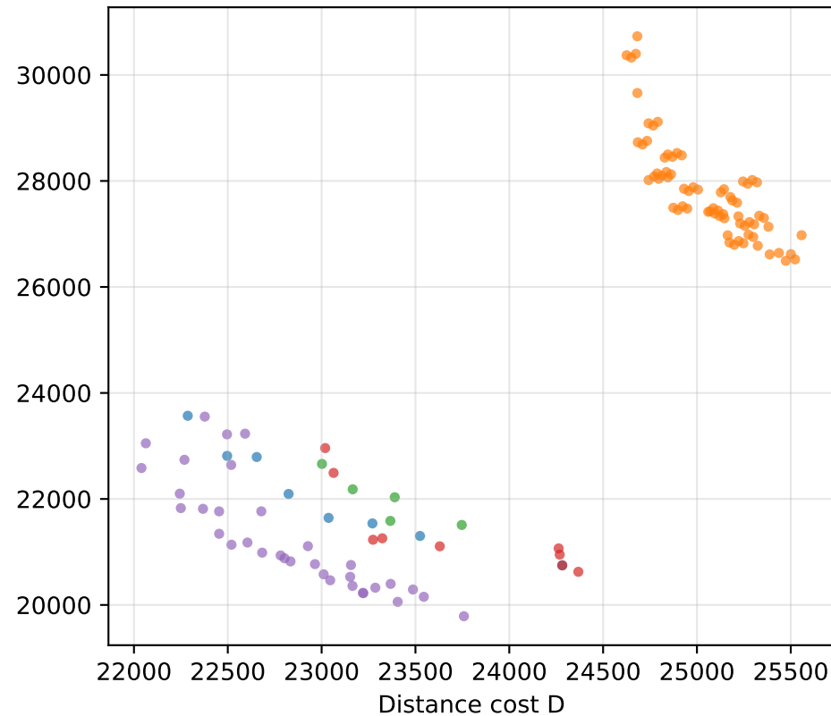
kroA100
