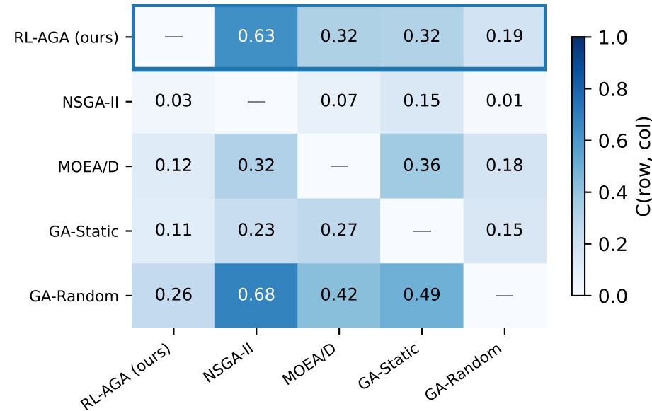
eil51
