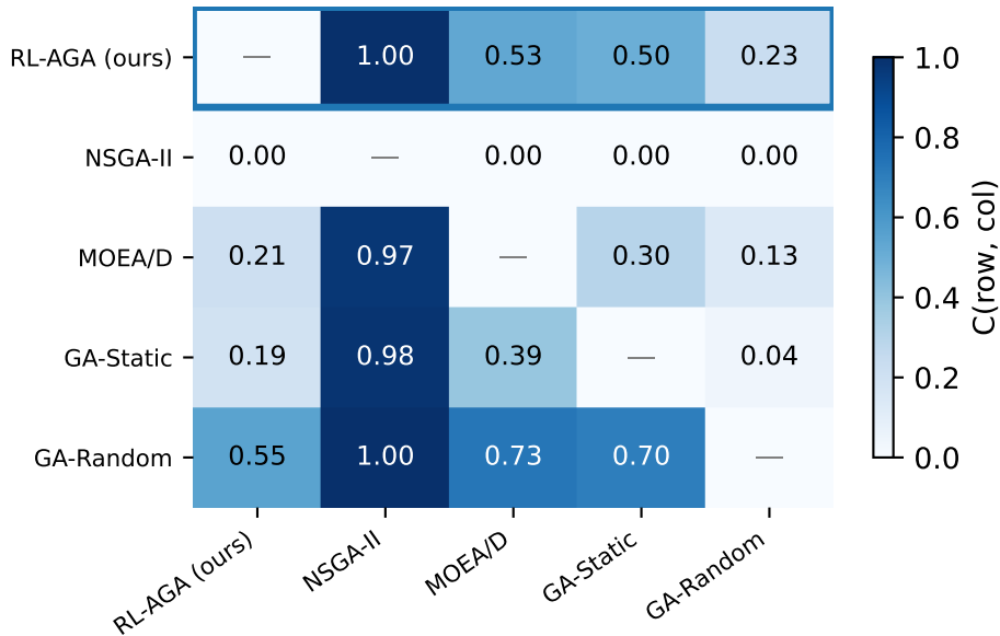
kroA100
