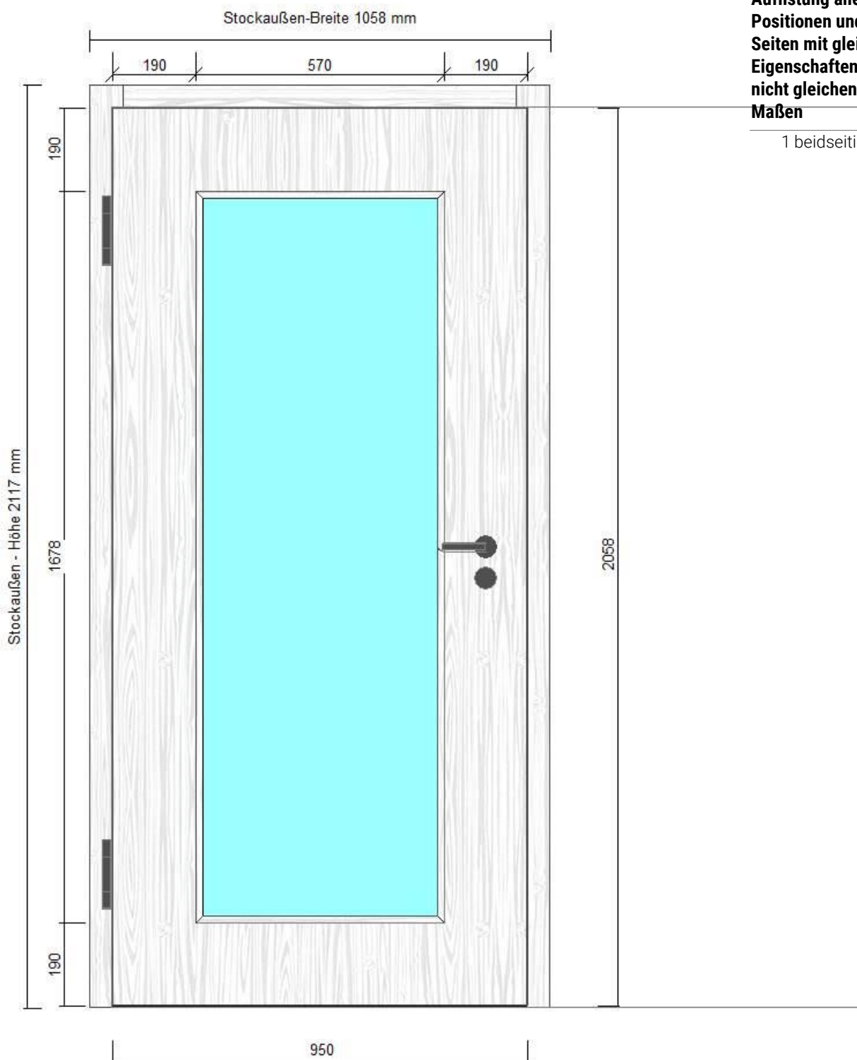
Türprofil
