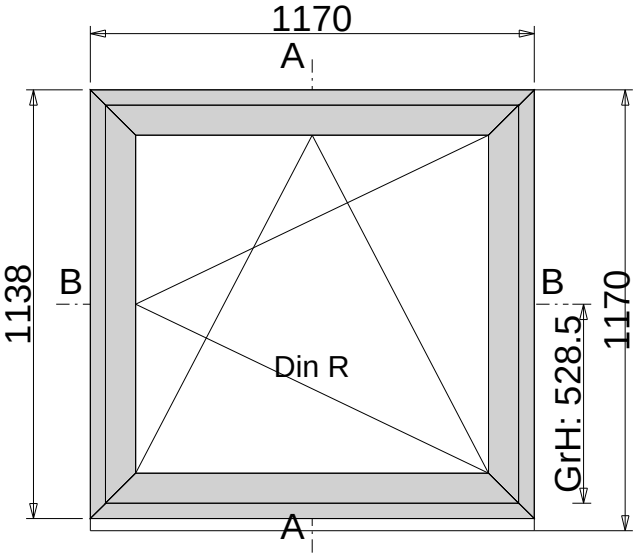
Ansicht von innen M 1:20
