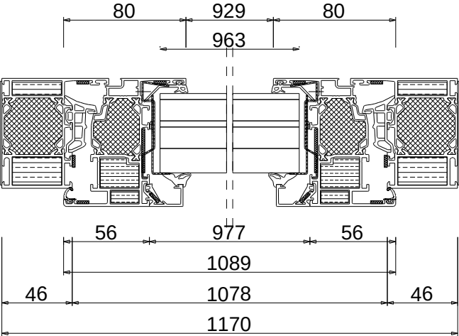
Schnitt B-B M 1:3.5
