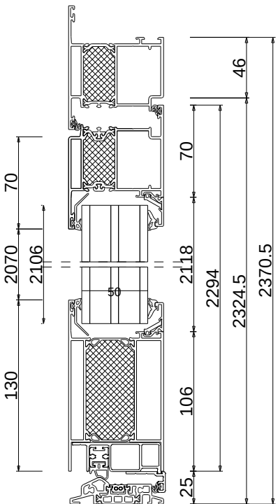
Schnitt A-A M 1:4
