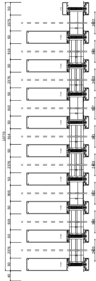
Schnitt B-B M 1:9
