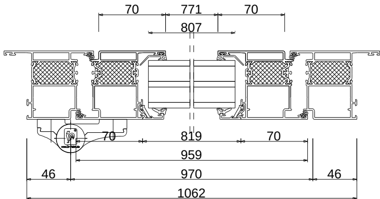
Schnitt B-B M 1:4
