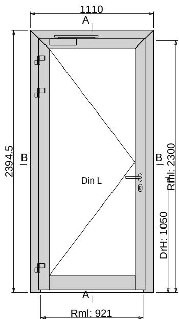
Ansicht von innen M 1:35
