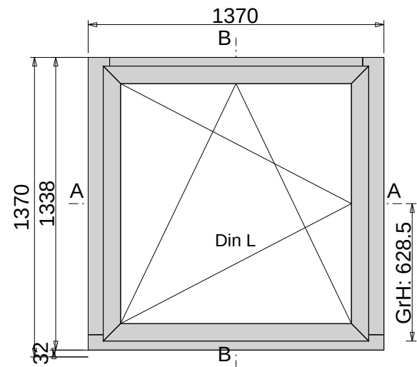
Ansicht von innen M 1:25
