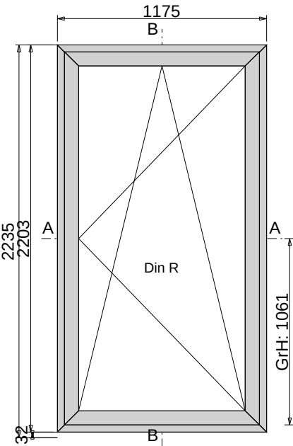
Ansicht von innen M 1:30
