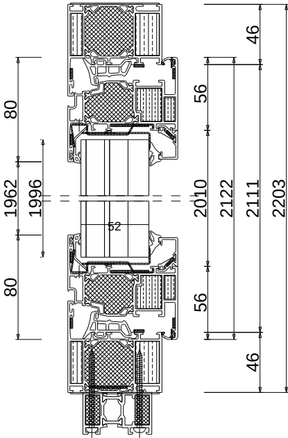
Schnitt B-B M 1:4
