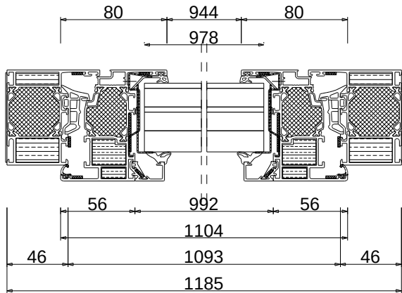
Schnitt A-A M 1:4
