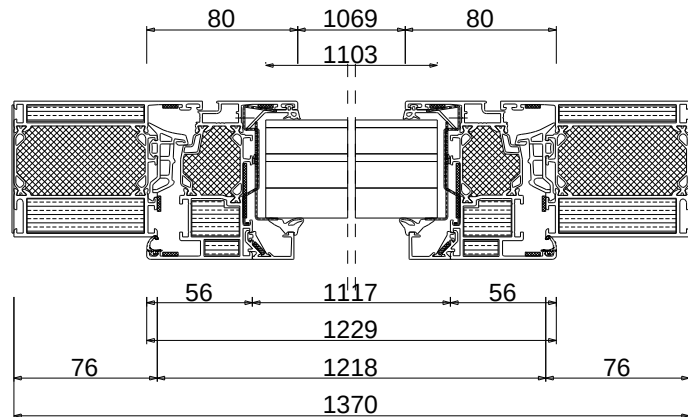
Schnitt A-A M 1:4
