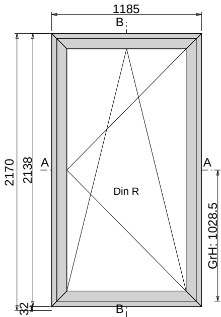
Ansicht von innen M 1:30
