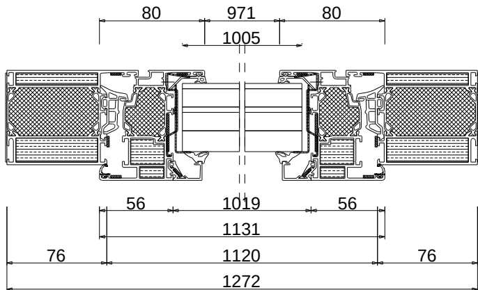
Schnitt A-A M 1:4
