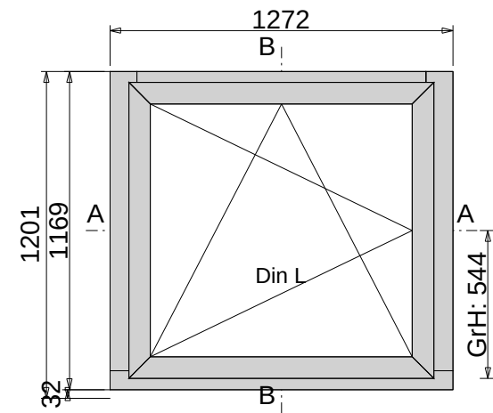
Ansicht von innen M 1:25
