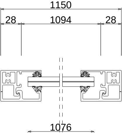
Schnitt A-A M 1:3
