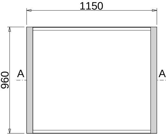
Ansicht von aussen M 1:20
