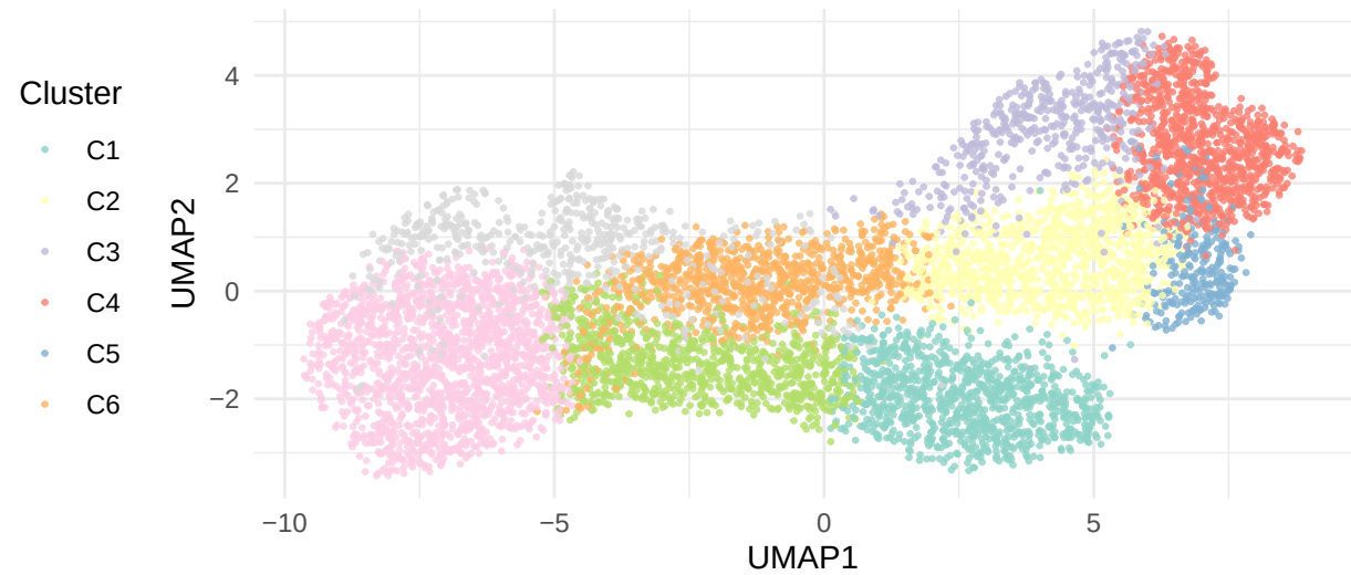
Alpha-Blend (k=6)
