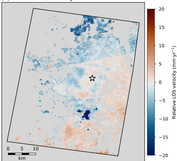
(a) Relative LOS velocity
