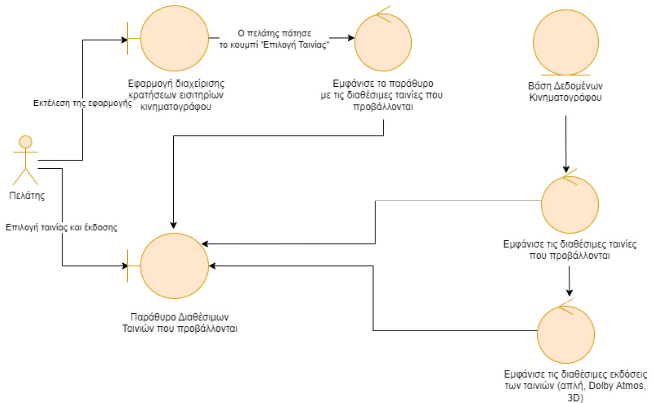
Εικόνα 5.1.3. Διάγραμμα Robustness της περίπτωσης χρήσης «Επιλογή ταινίας»
