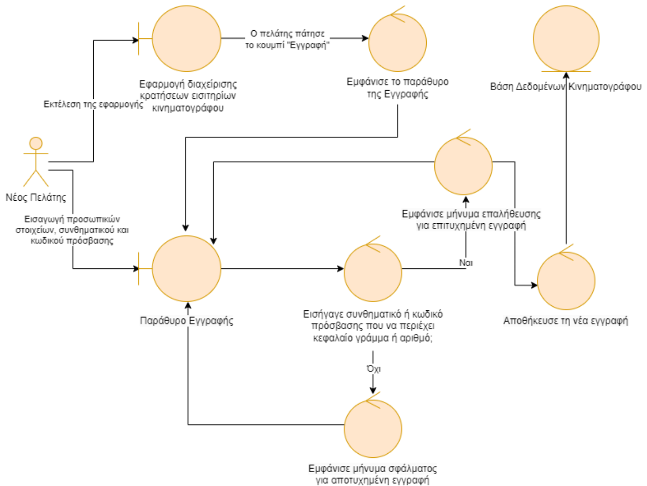
Εικόνα 5.1.1. Διάγραμμα Robustness της περίπτωσης χρήσης «Εγγραφή»
