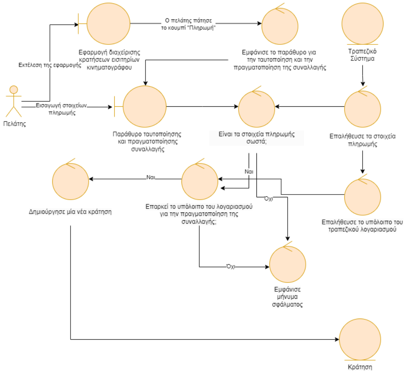
Εικόνα 5.1.7. Διάγραμμα Robustness της περίπτωσης χρήσης «Πληρωμή»
