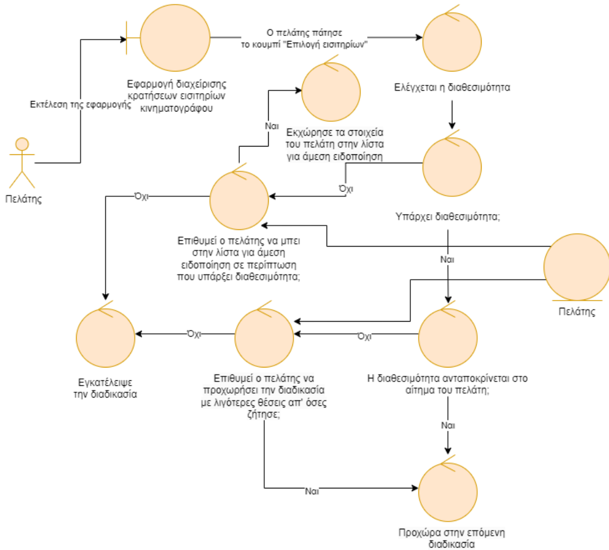
Εικόνα 5.1.6. Διάγραμμα Robustness της περίπτωσης χρήσης «Έλεγχος διαθεσιμότητας»
