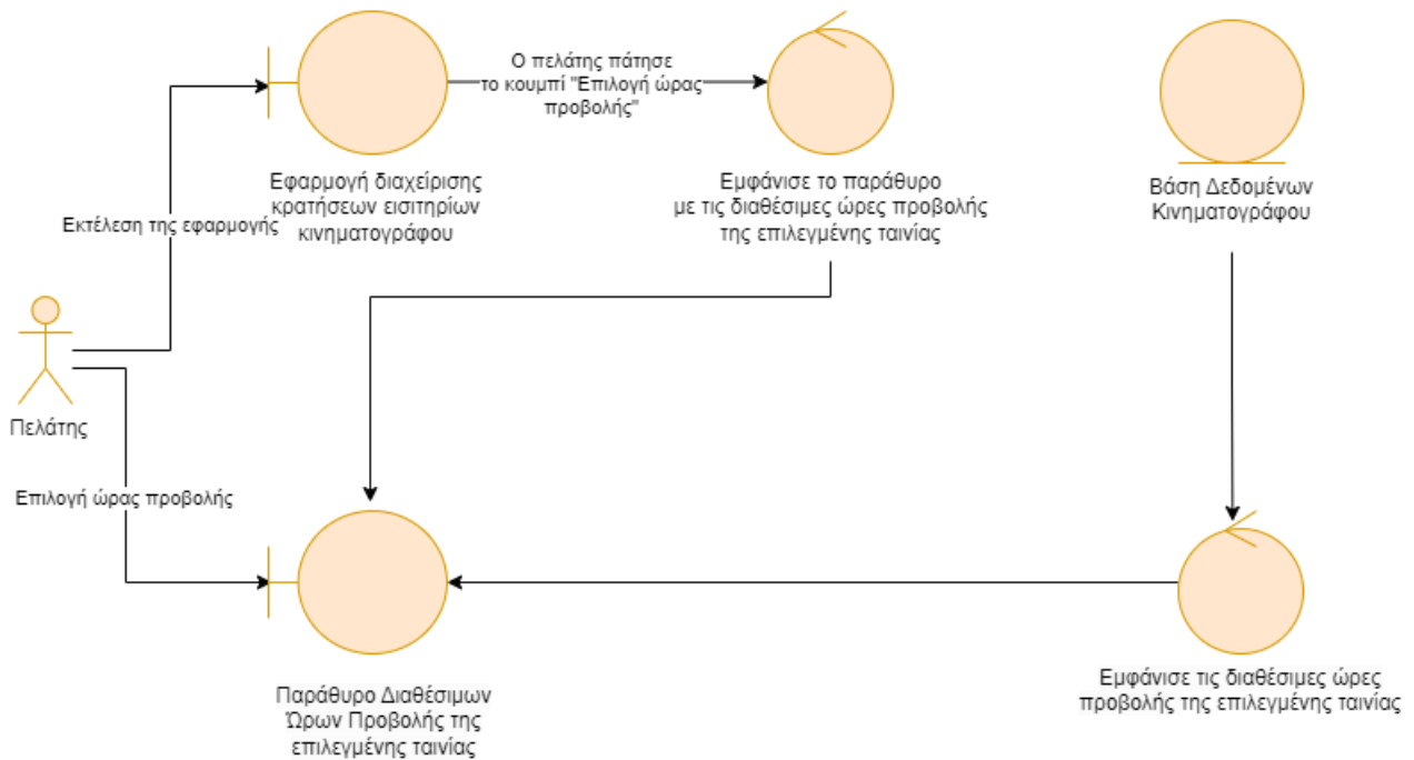
Εικόνα 5.1.4. Διάγραμμα Robustness της περίπτωσης χρήσης «Επιλογή ώρας προβολής»
