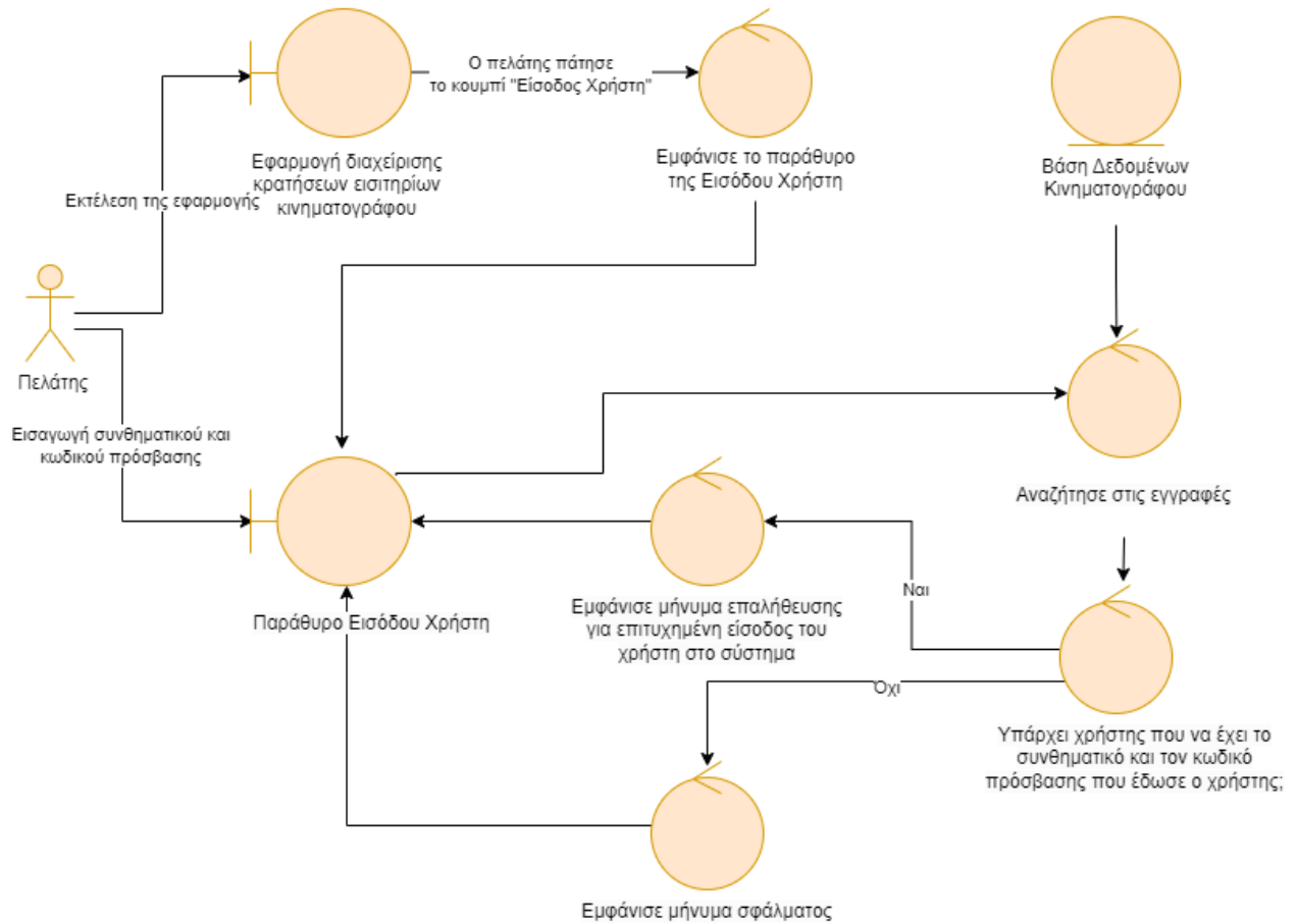
Εικόνα 5.1.2. Διάγραμμα Robustness της περίπτωσης χρήσης «Είσοδος Χρήστη»
