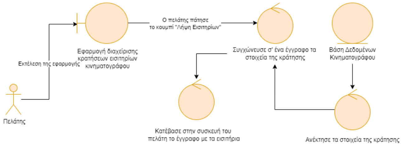
Εικόνα 5.1.9. Διάγραμμα Robustness της περίπτωσης χρήσης «Λήψη Εισιτηρίων»
