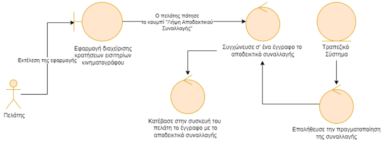
Εικόνα 5.1.8. Διάγραμμα Robustness της περίπτωσης χρήσης «Λήψη Αποδεικτικού Συναλλαγής»
